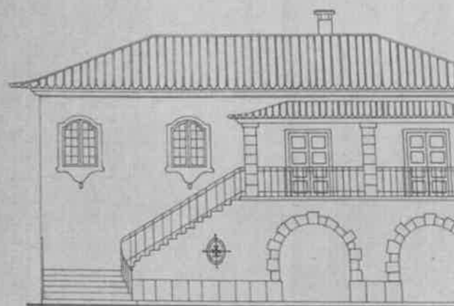
ALÇADO PRINCIPAL
