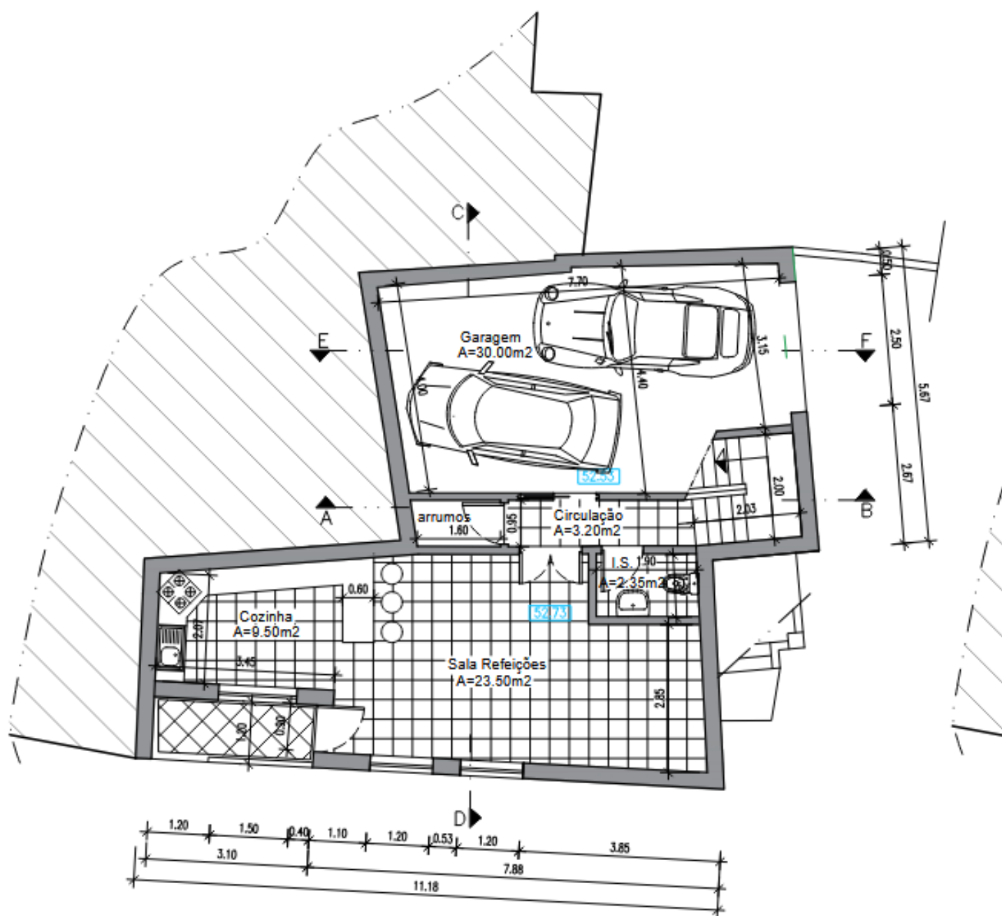
PLANTA DA CAVE
