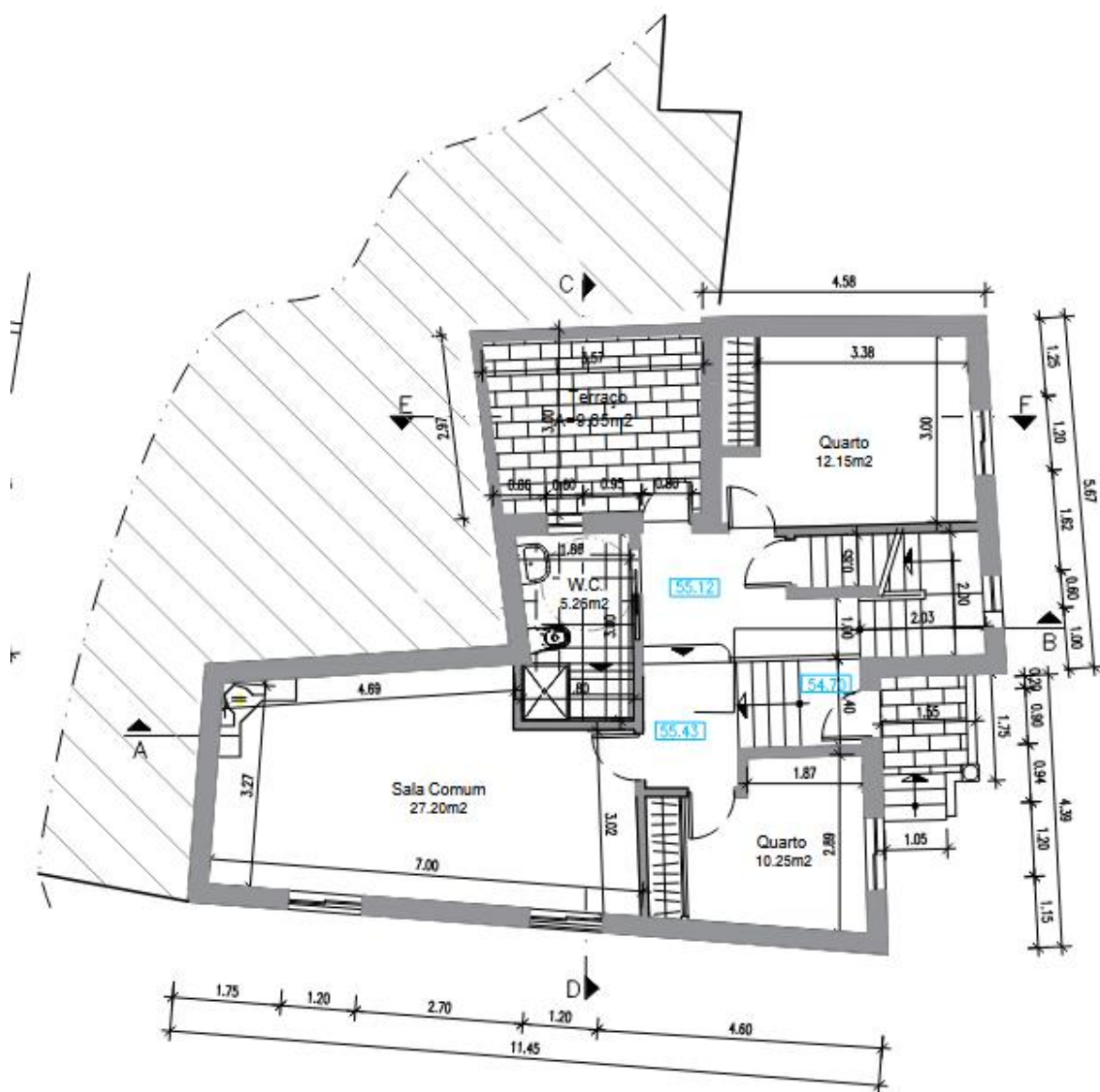
PLANTA DO R/CHÃO
