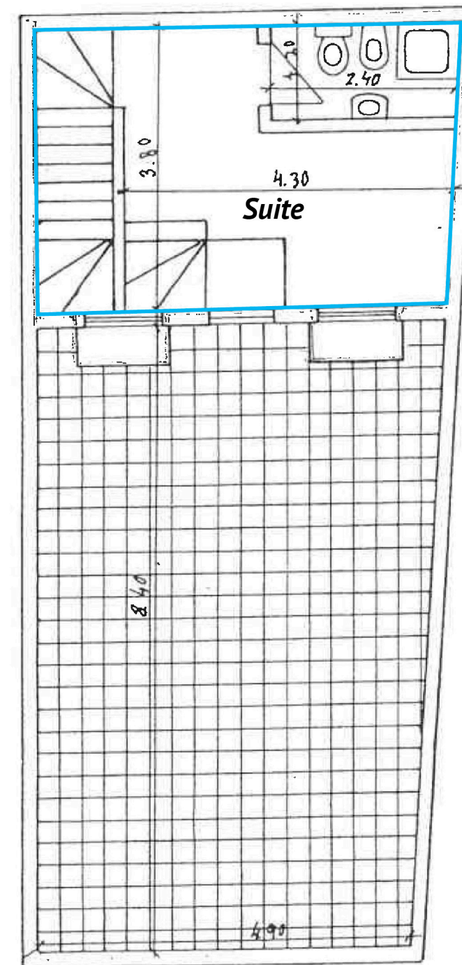
1.º andar
