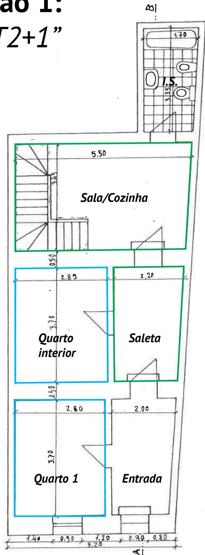
Rés-do-chão
