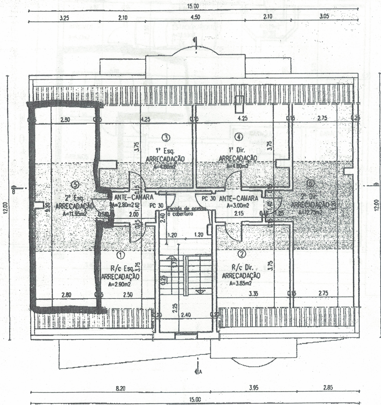
Planta do sótão
