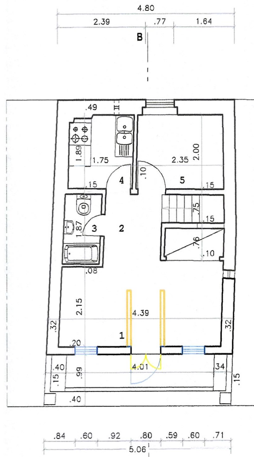
Planta do 4º andar
