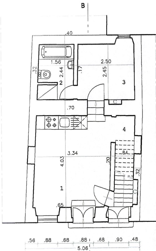
Planta do r/chão
