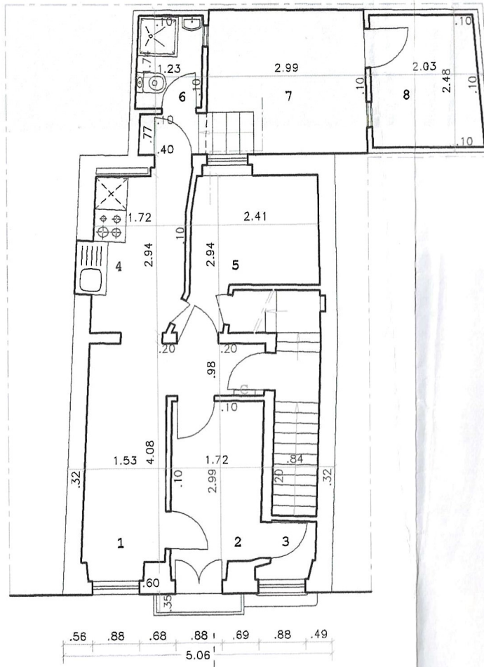
Planta do 1º andar
