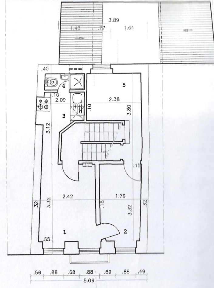
Planta do 2º andar
