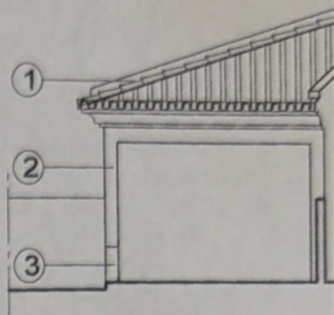
ALÇADO NASCENTE
