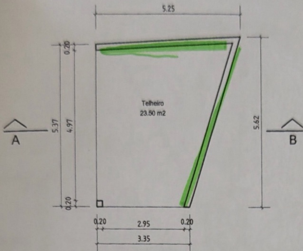
PLANTA
