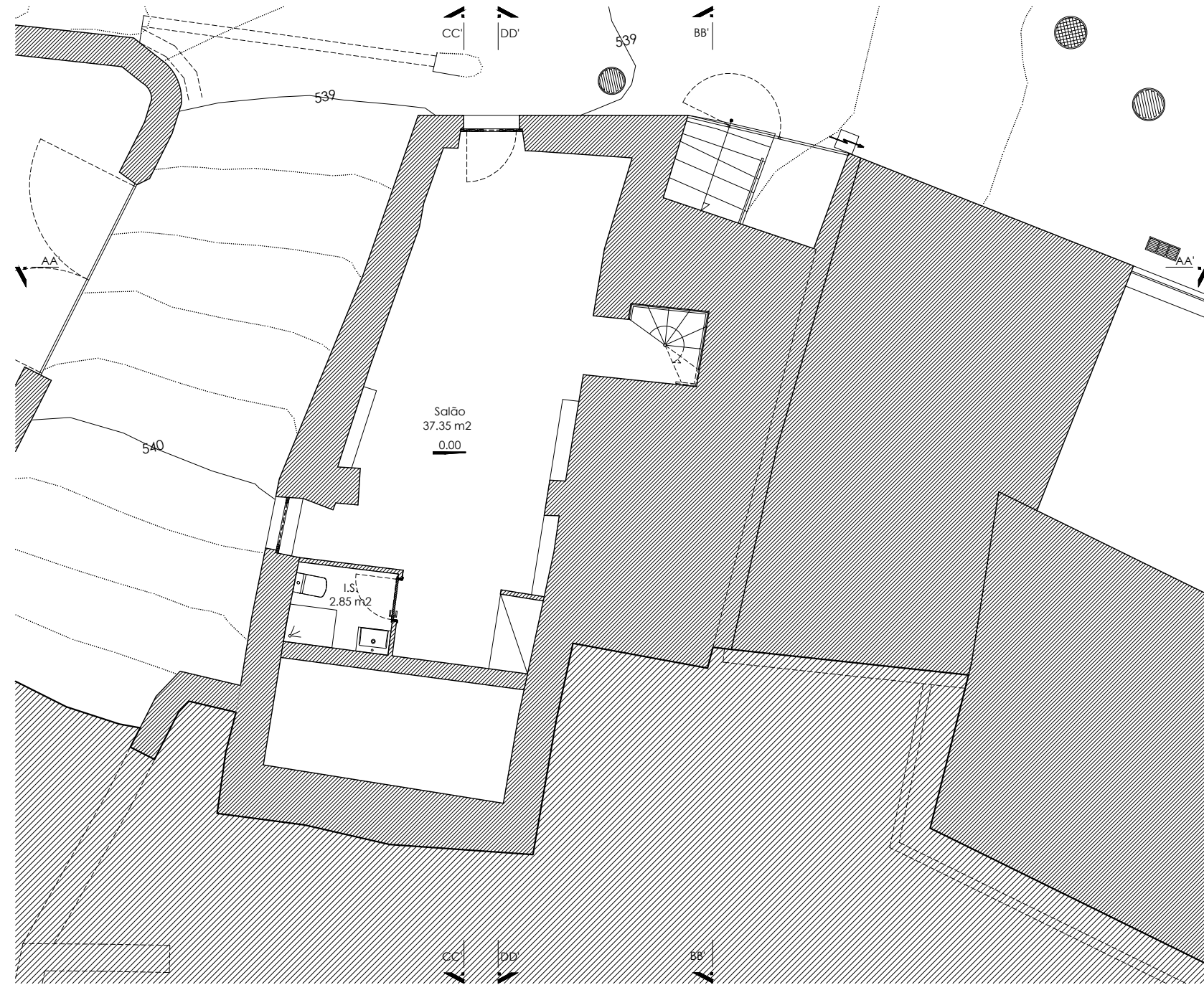
PLANTA PISO 0
