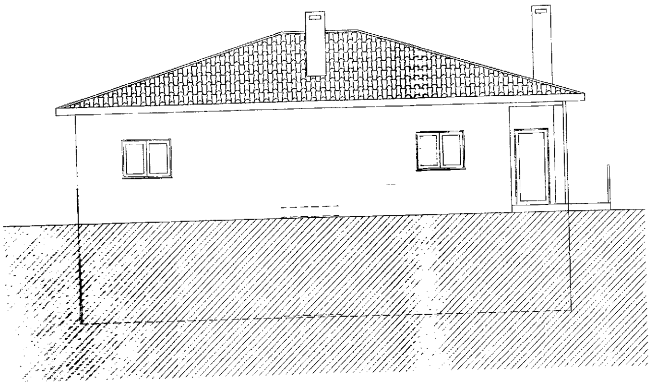
ALÇADO LAT. ESQUERDO
