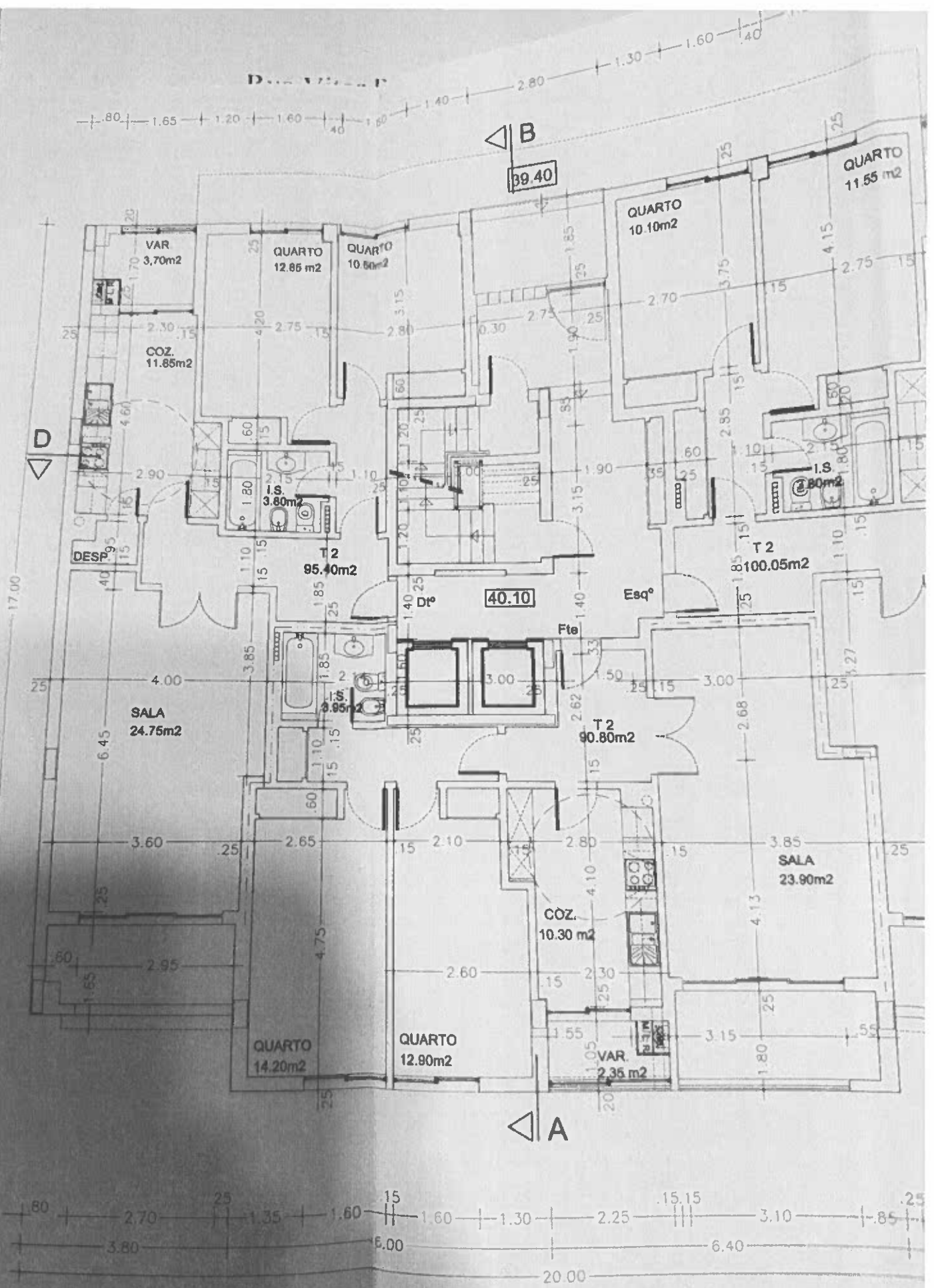
PLANTA DO BLOCO (PISO 0)
