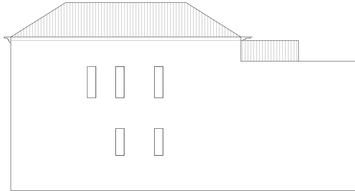
ALÇADO POENTE
