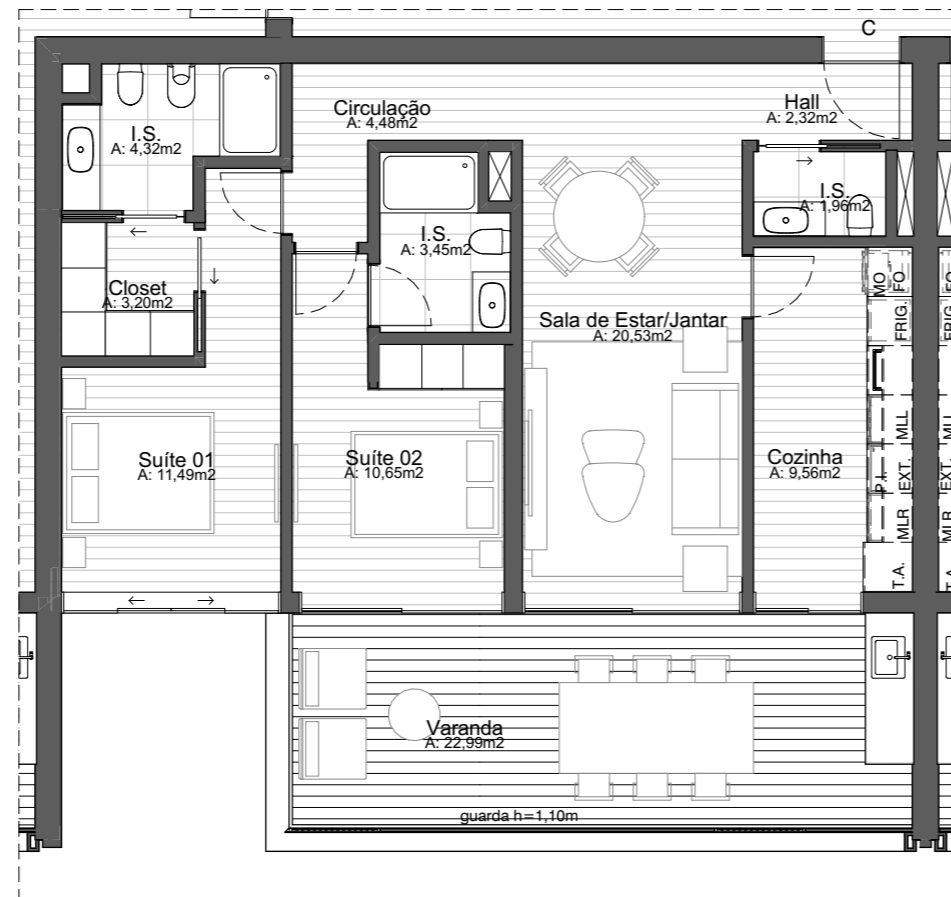
PLANTA - APARTAMENTO 2C 1:100
