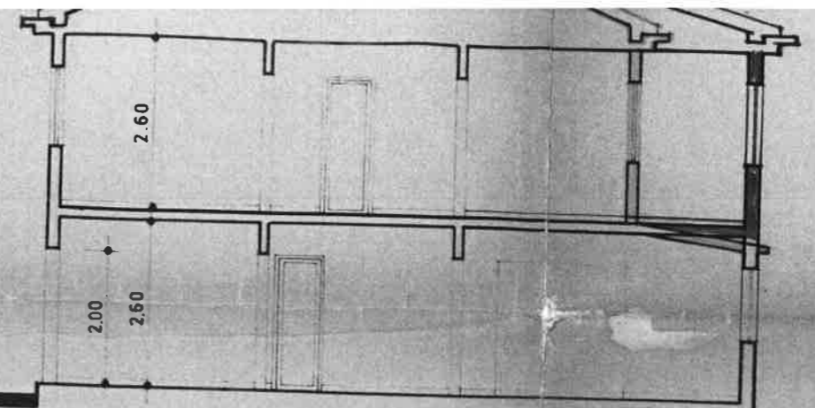
CORTE A:B
