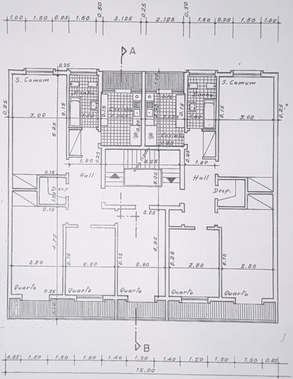
PLANTA DOS ANDARES
