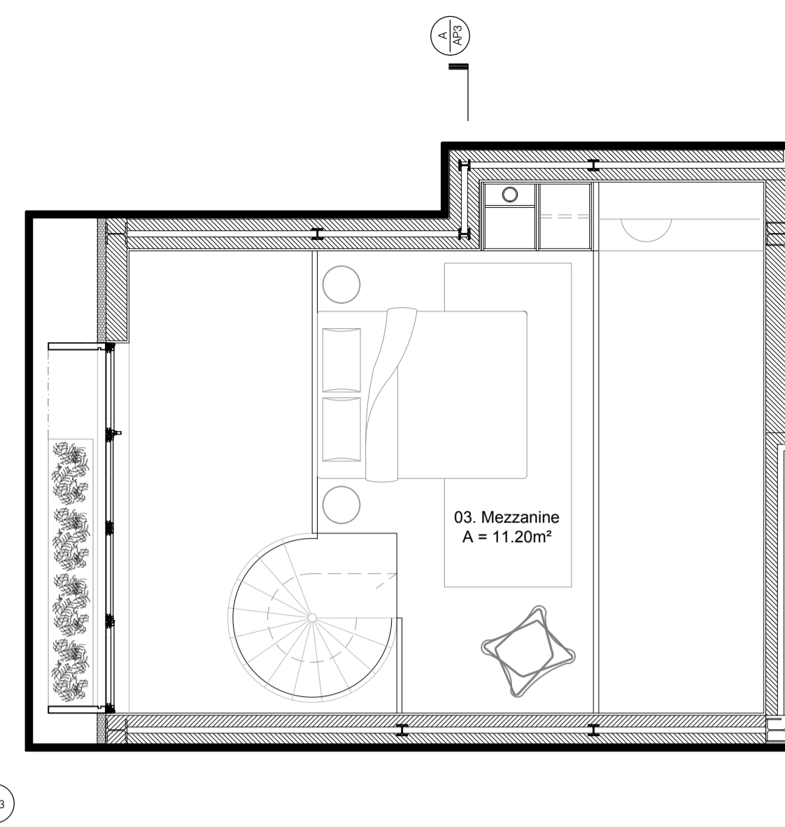
Planta Piso 1
