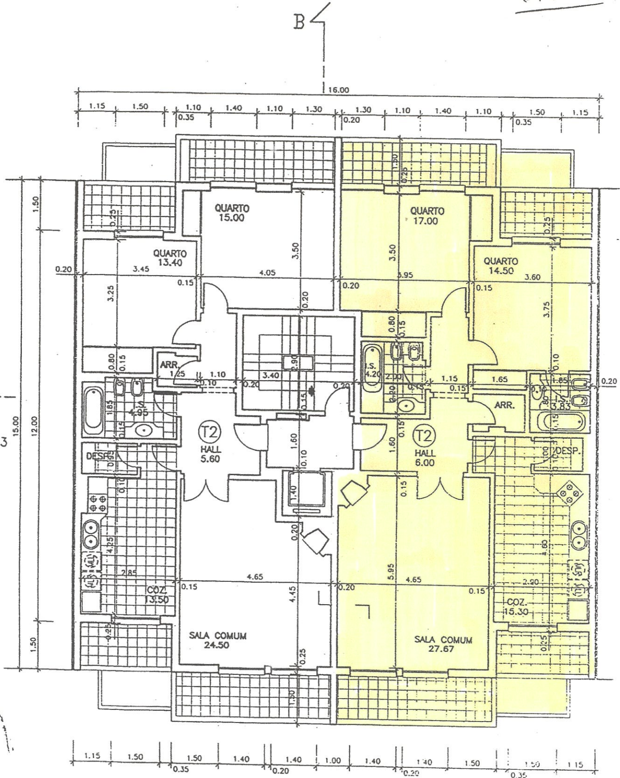
PLANTA DO ANDAR RECUADO
