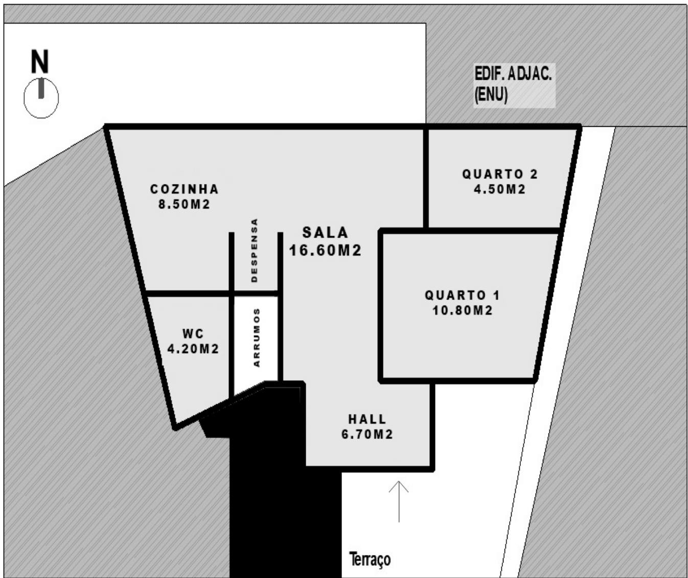
Planta (1º Andar)
