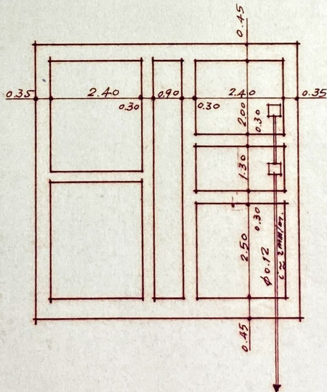
FUNDAÇÕES
