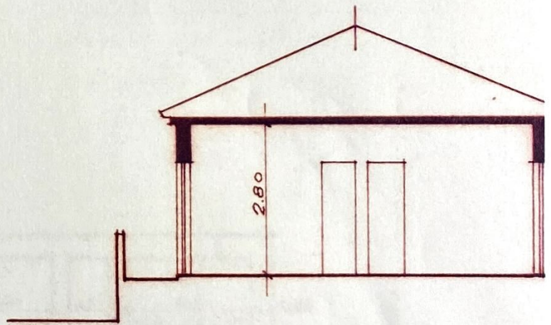
CORTE A-B
