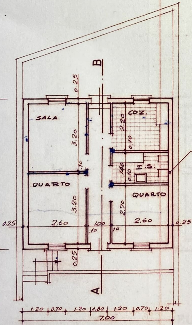
PLANTA
