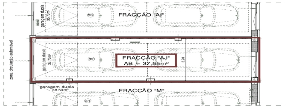
CAVE ( PISO 0 ) ESCALA: 1/100
