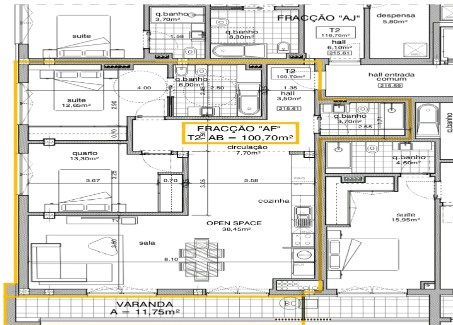
6º ANDAR ( PISO 7 ) ESCALA: 1/100
