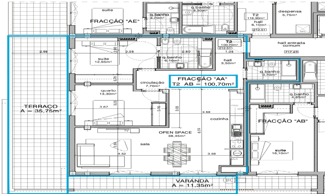
5º ANDAR ( PISO 6 ) ESCALA: 1/100
