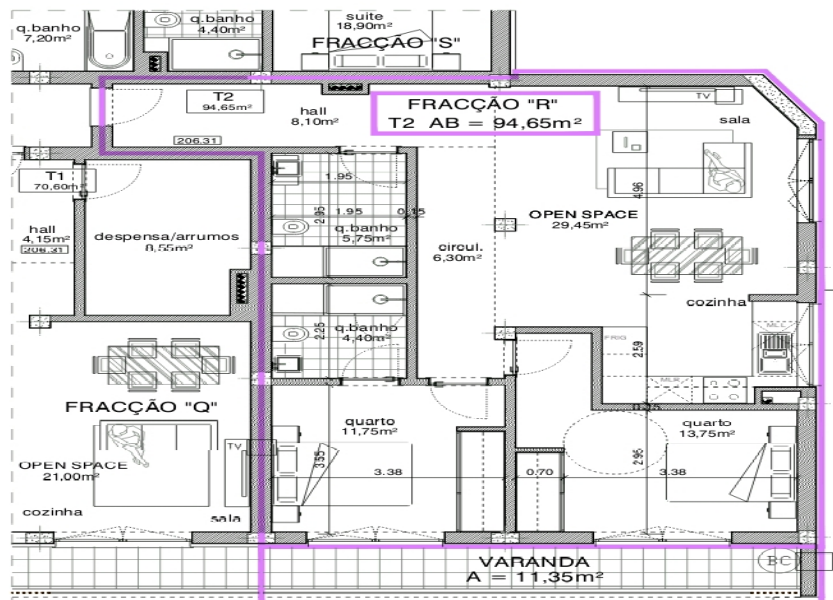
3º ANDAR ( PISO 4 ) ESCALA: 1/100
