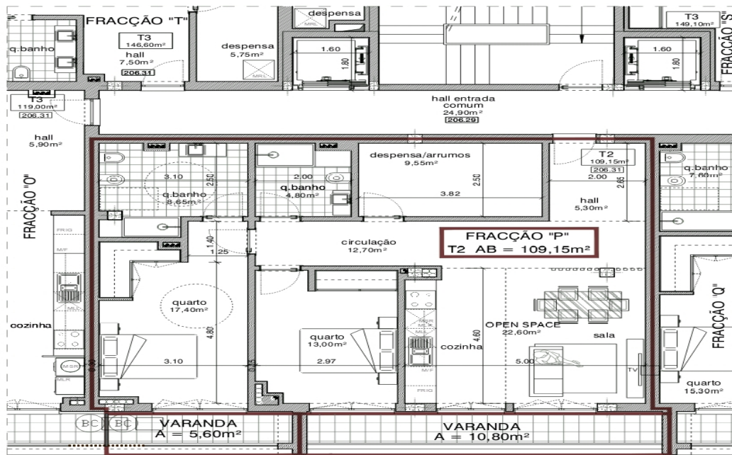
3º ANDAR ( PISO 4 ) ESCALA: 1/100
