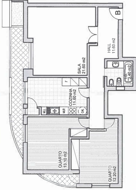
PLANTA DO R/CHÃO - FRACÇÃO B
