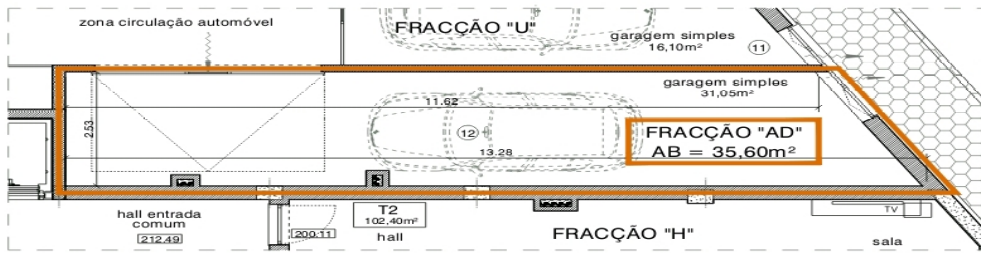
1º ANDAR ( PISO 2 ) ESCALA: 1/100
