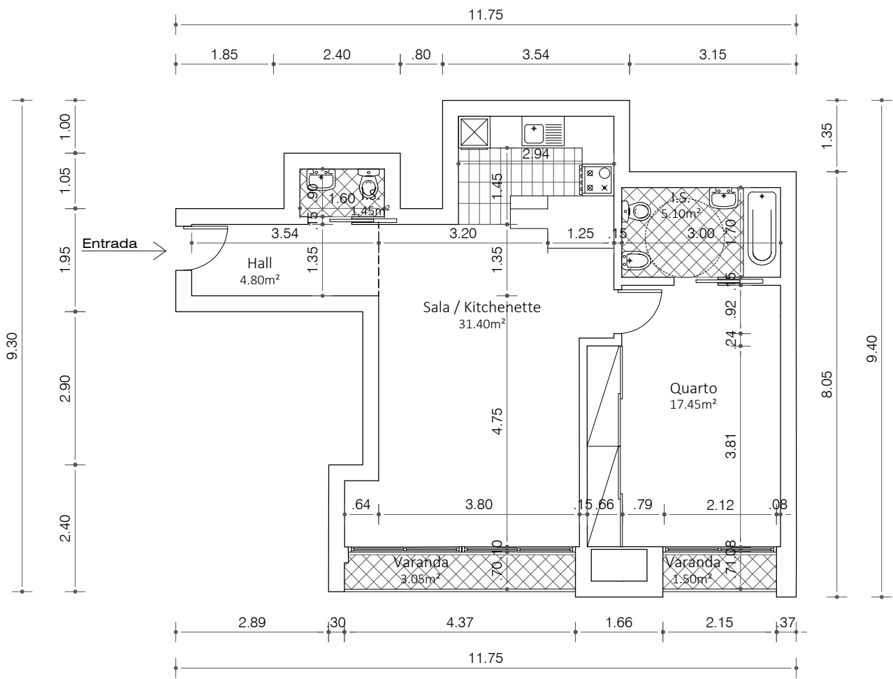
Planta Baixa C - Piso 6 ESC. 1/100
