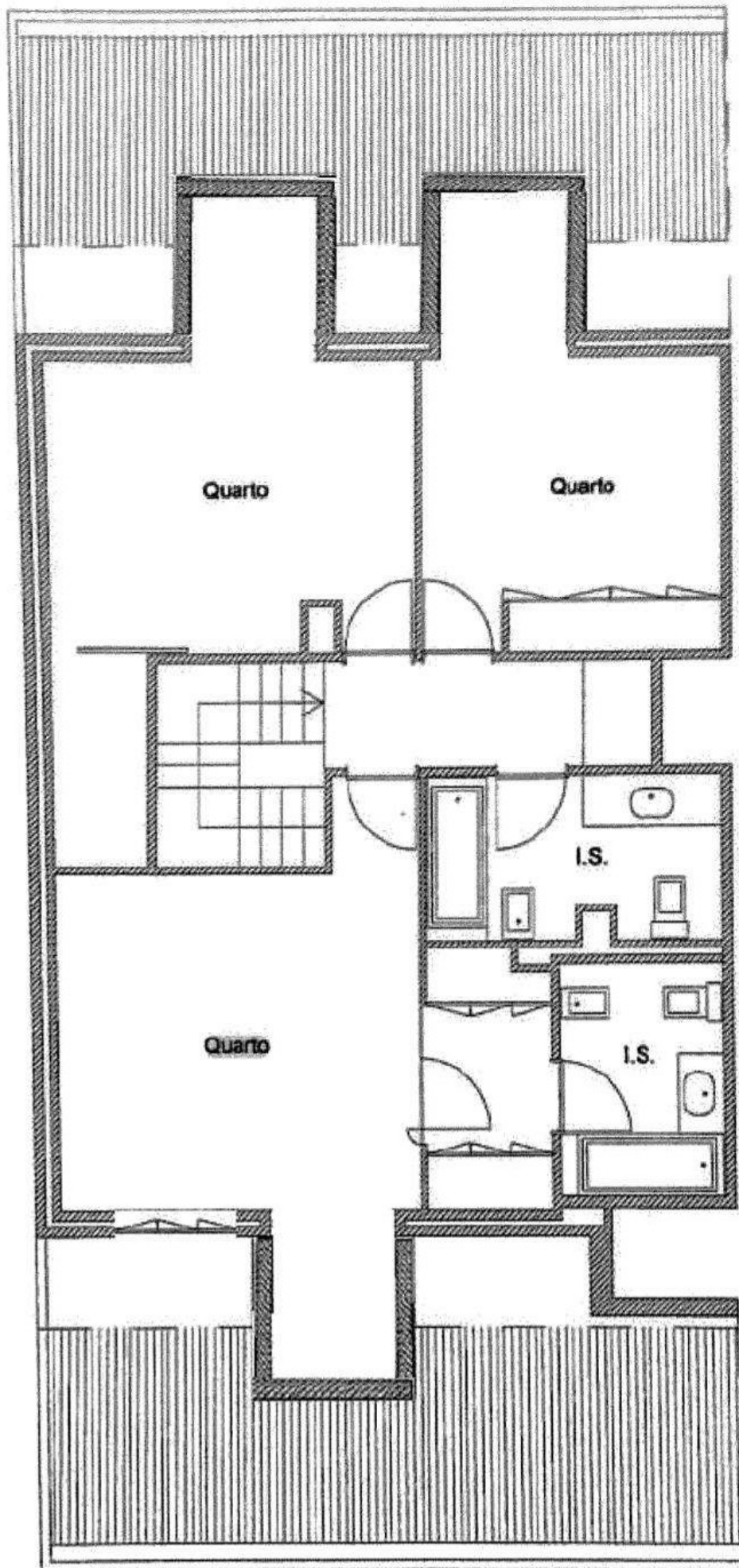
PLANTA SIMPLIFICADA DA HABITAÇÃO FRACÇÃO AUTÓNOMA "J" PLANTA DO VÃO DA COBERTURA
