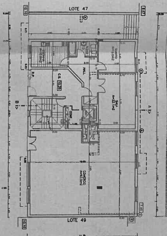
PLANTA DO R/C
