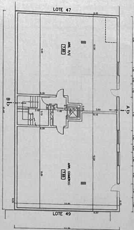
PLANTA DA CAVE
