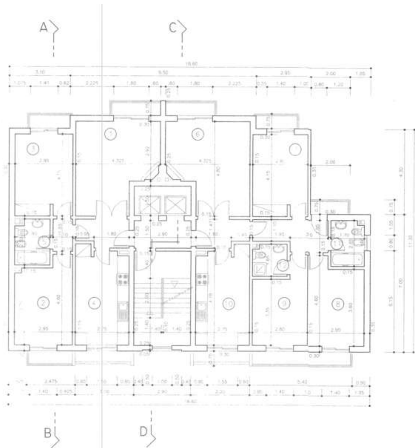
PLANTA DOS PISOS 2 a12
