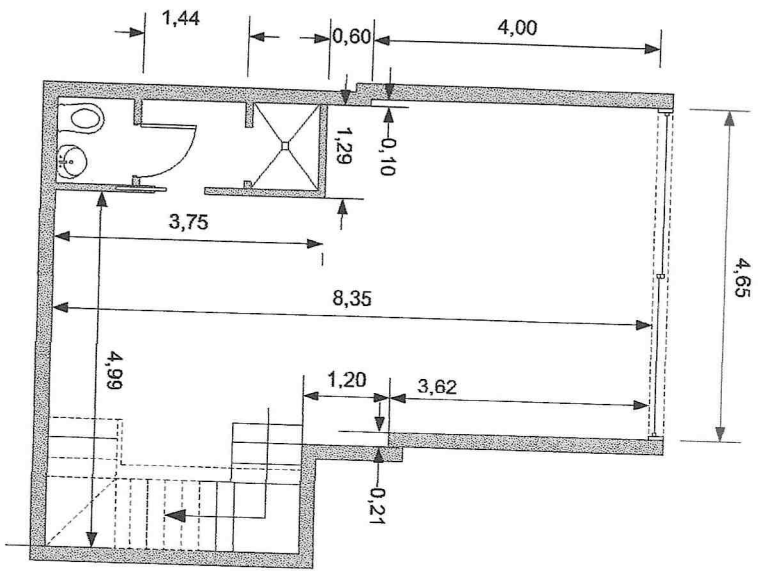
CAVE - PÉ DIREITO COM 3,00 MT
