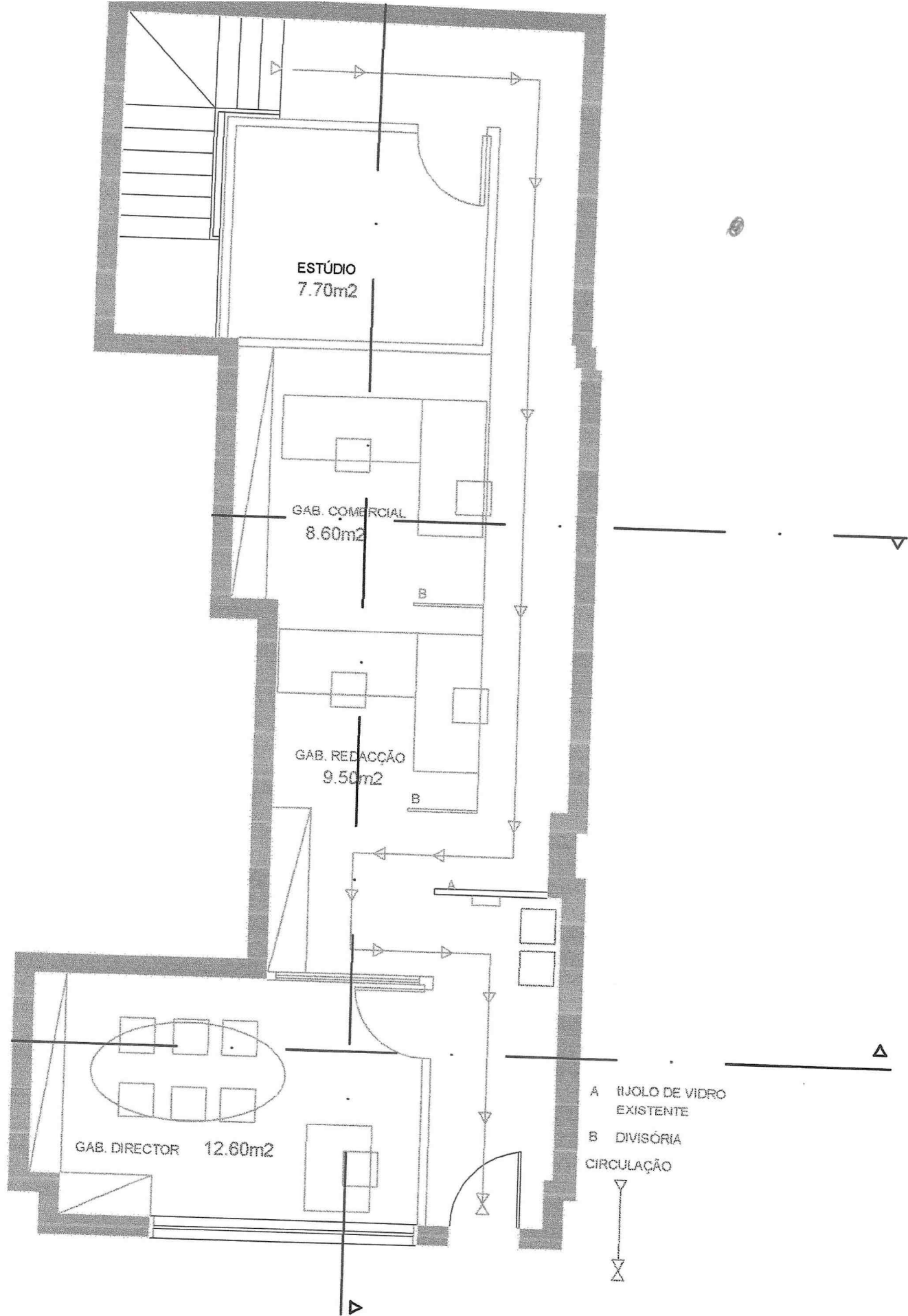
PLANTA DE MOBILIÁRIO E CIRCULAÇÃO
