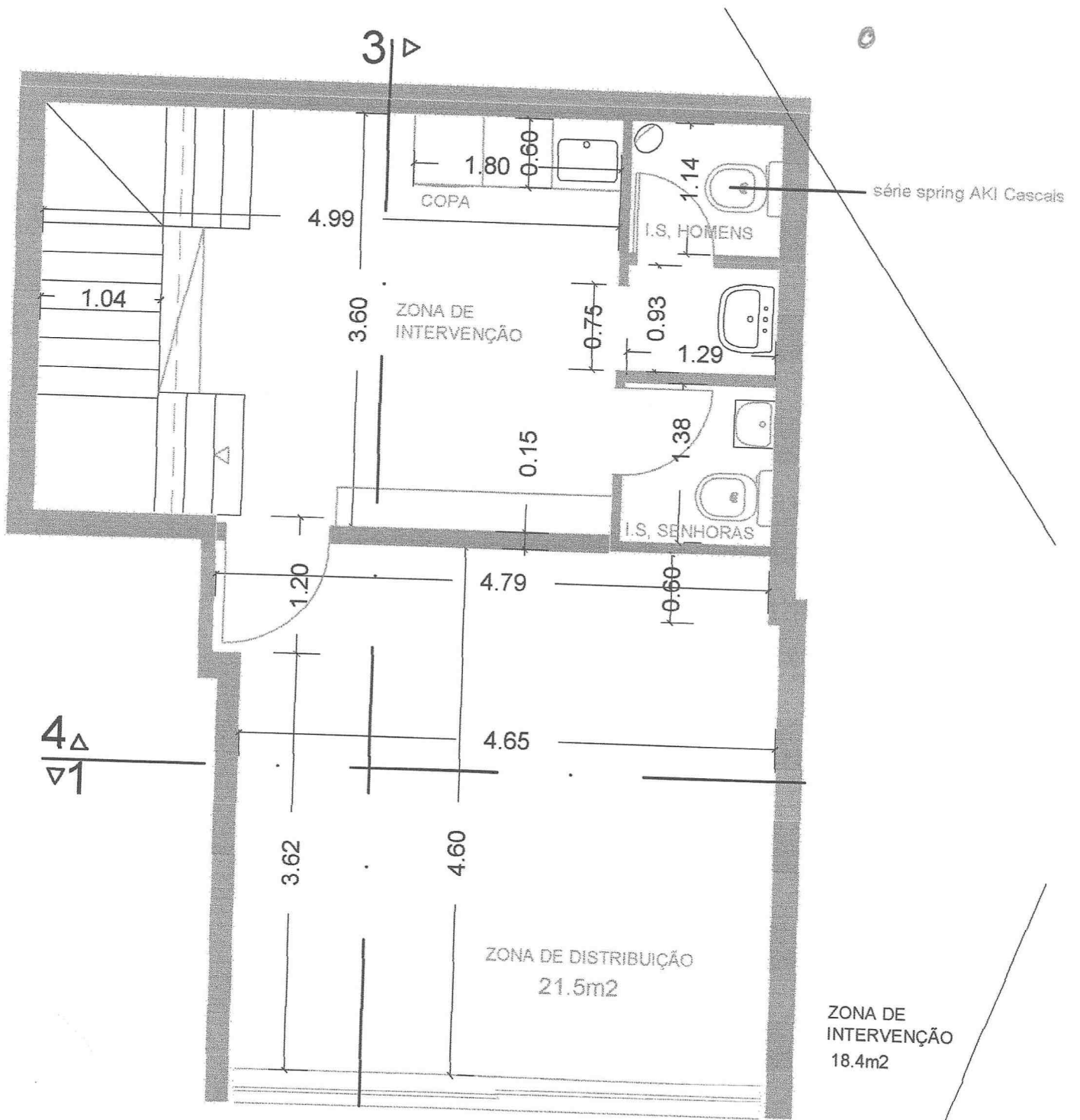
PLANTA DA CAVE
