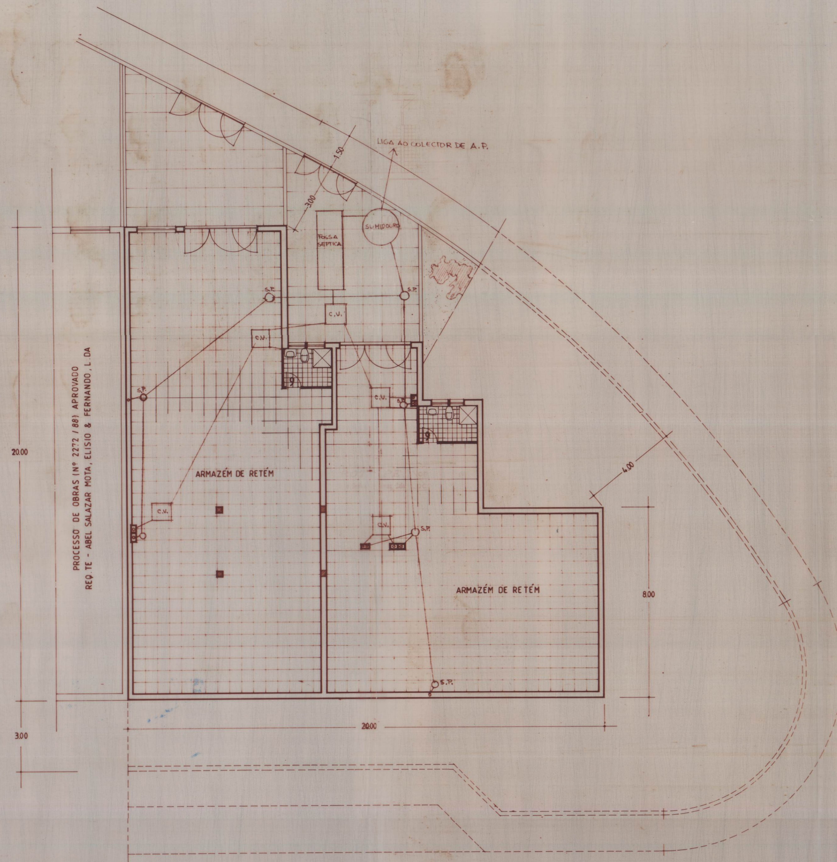
PLANTA DA SUB-CAVE
