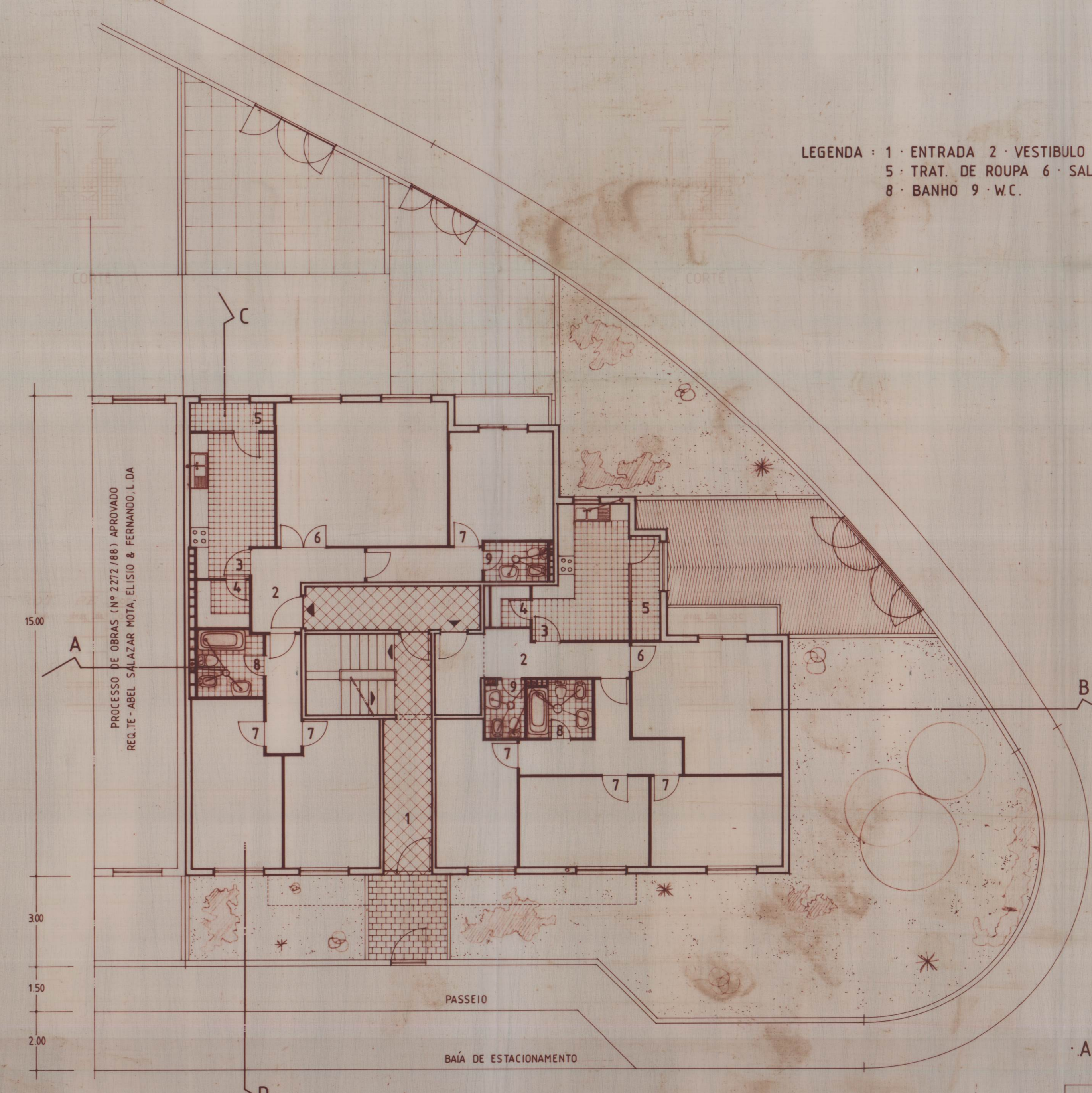
PLANTA DO RÉS-DO-CHÃO
