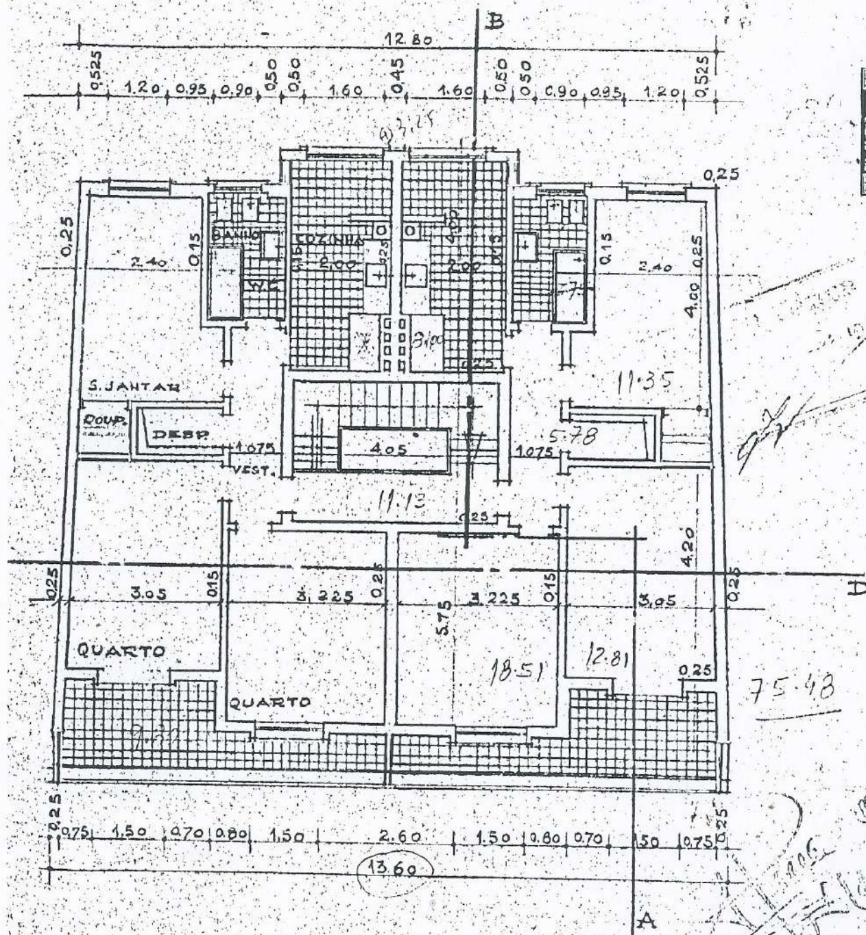
PLANTA DOS ANDARÉS
