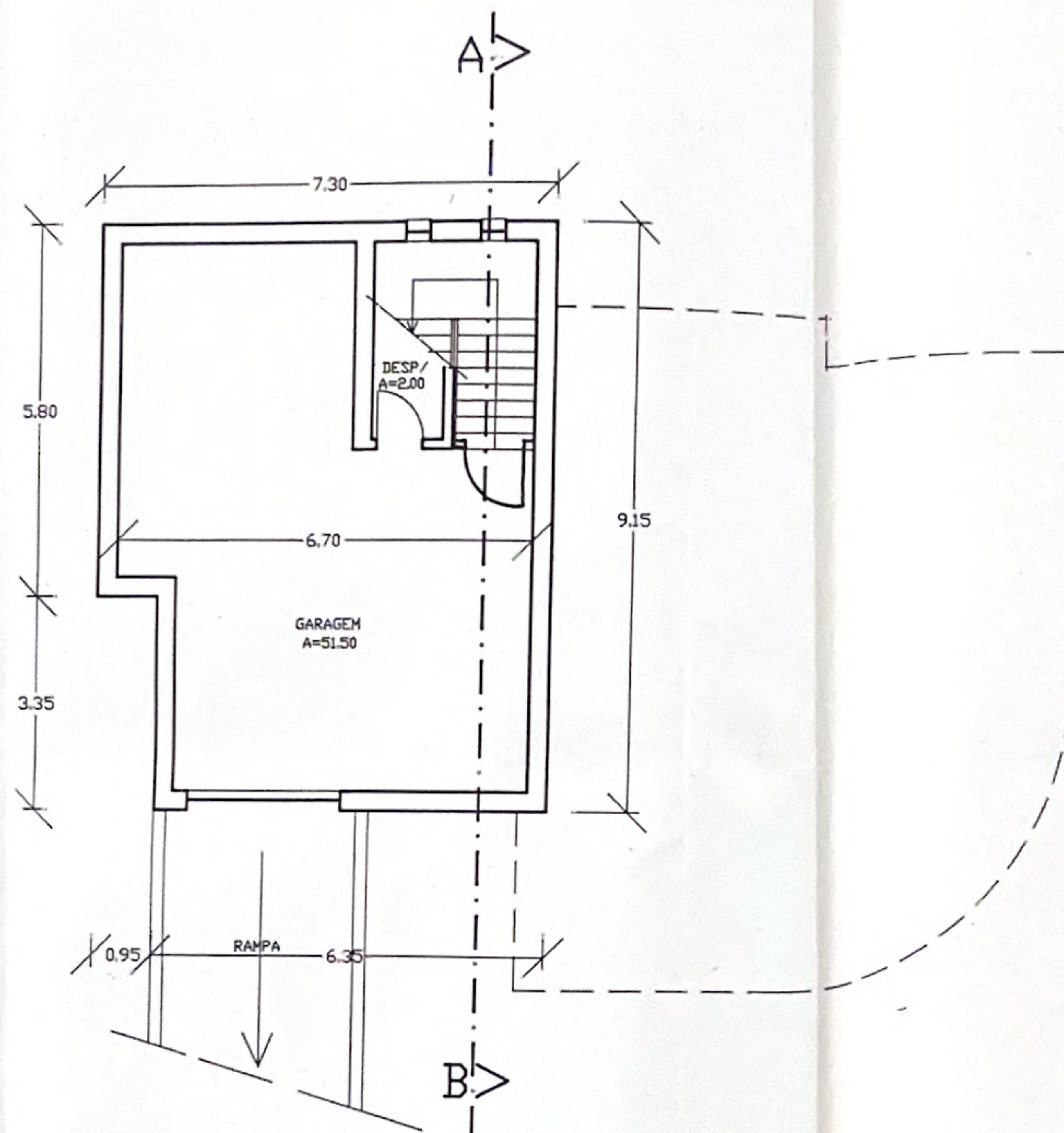
PLANTA DA CAVE
