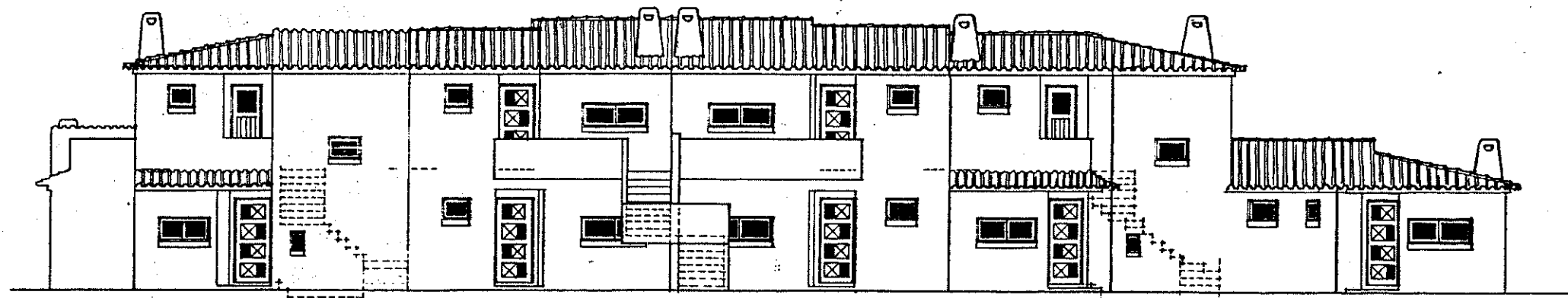
ALÇADO NORTE
