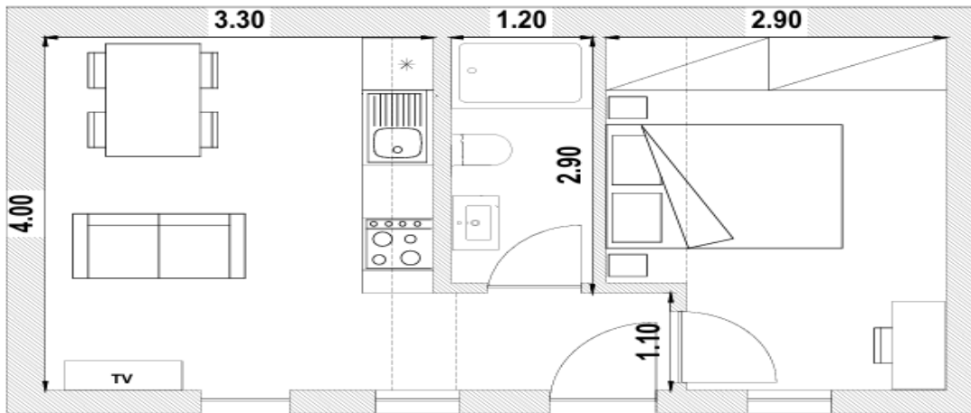
Planta cotada
