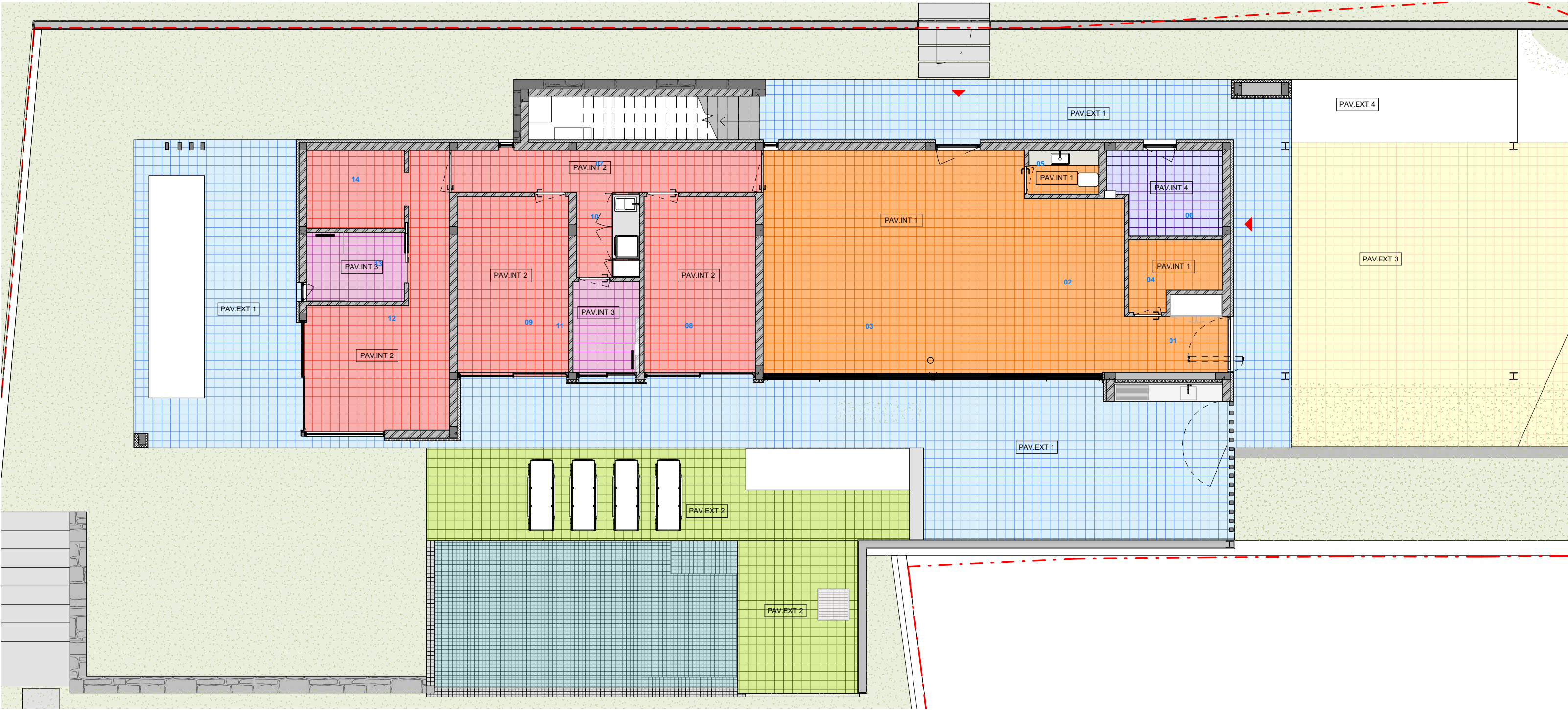
PLANTA PISO 00 ESCALA: 1 : 100
