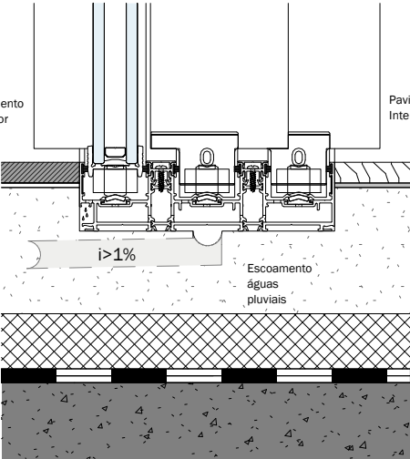
SOLEIRA 5 - VÃO OS TRIPLO
