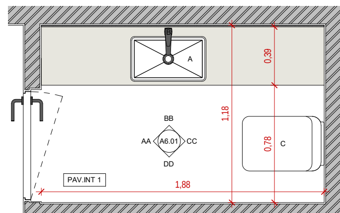
I.S. SOCIAL - PLANTA ESCALA: 1 : 25
