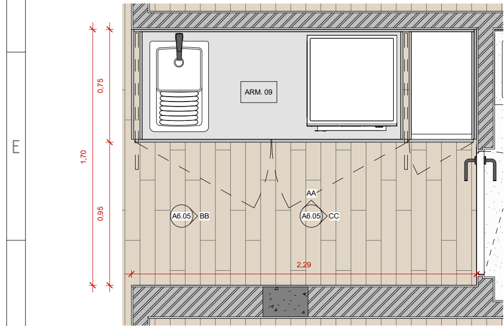
LAVANDARIA - PLANTA
