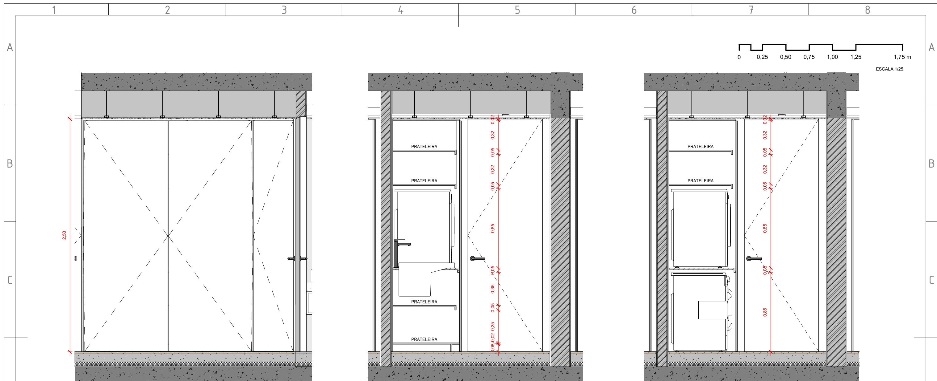
LAVANDARIA - CORTE AA
