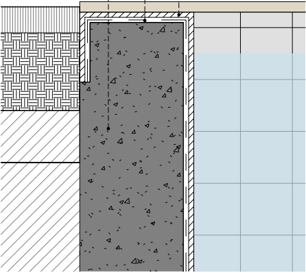
Elevation 1 - c - Callout 1 ESCALA: 1 : 10
