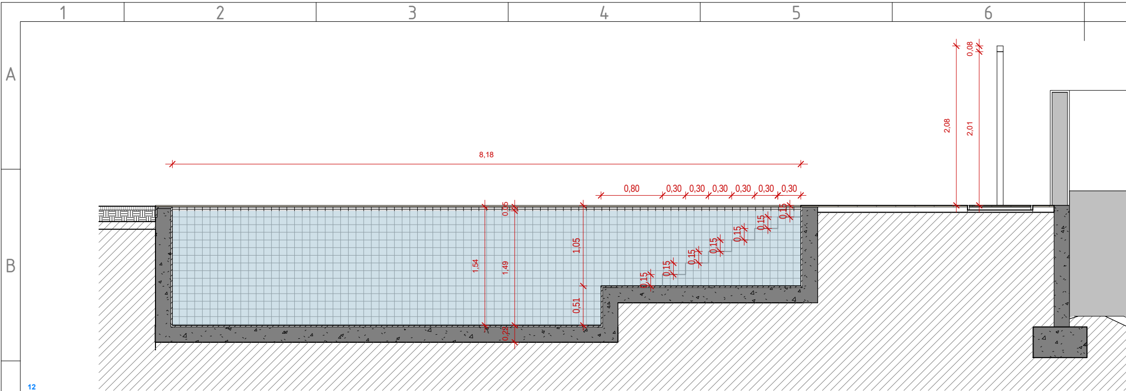
CORTE LONGITUDINAL ESCALA: 1 : 50
