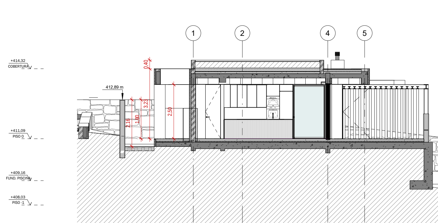
CORTE DD ESCALA: 1 : 100
