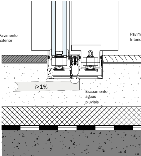
SOLEIRA 4 - VÃO OS DUPLO
