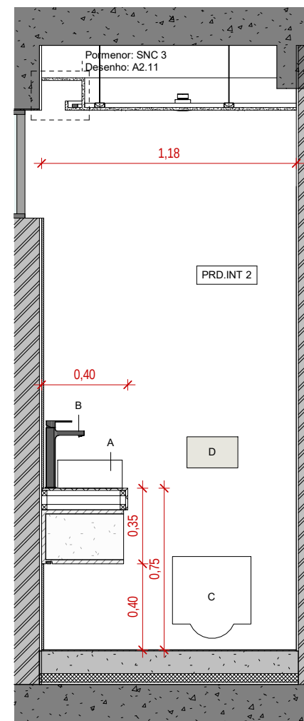
I.S. SOCIAL - CORTE CC ESCALA: 1 : 25
