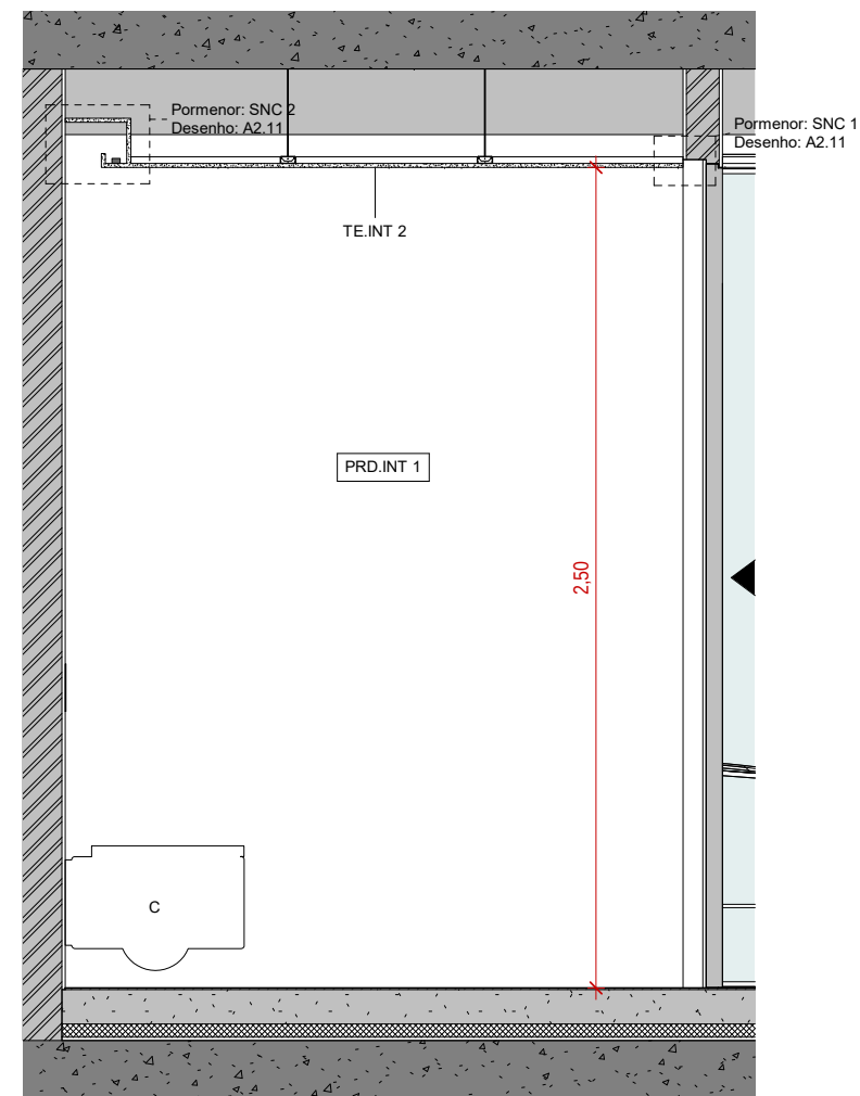
I.S. SOCIAL - CORTE DD ESCALA: 1 : 25
