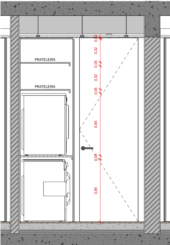
LAVANDARIA - CORTE CC
