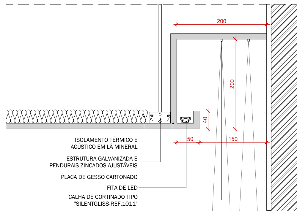
SNC 4 - SANCA DE LUZ COM CORTINADO ESCALA: 1 : 5
