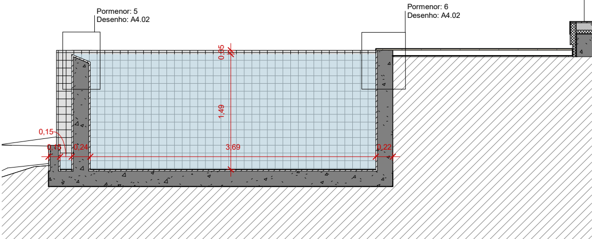
CORTE TRANSVERSAL ESCALA: 1 : 50
