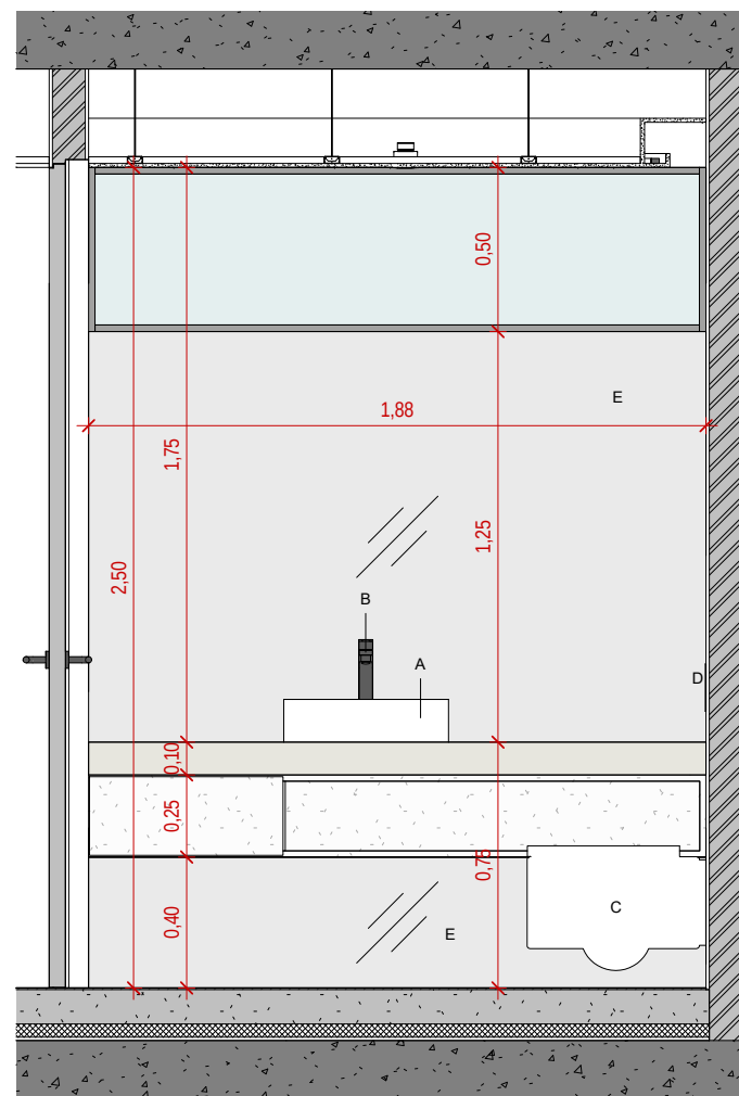
I.S. SOCIAL - CORTE BB ESCALA: 1 : 25
