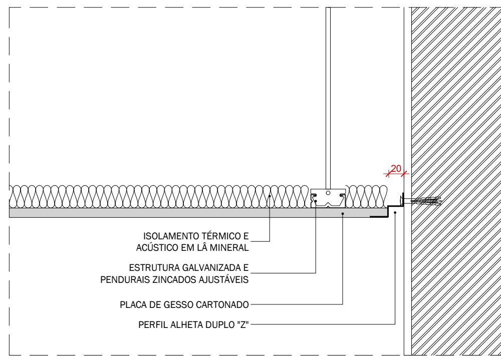
SNC 1 - SANCA DE TECTOS - DUPLO Z ESCALA: 1 : 5
