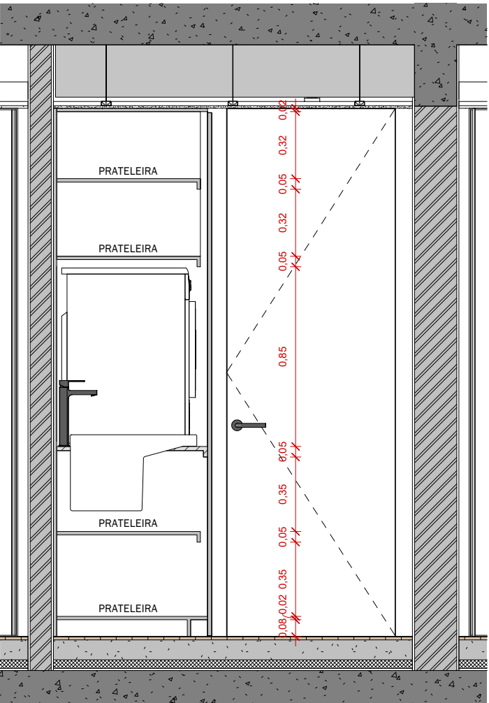
LAVANDARIA - CORTE BB
