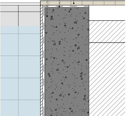
Elevation 1 - c - Callout 3 ESCALA: 1 : 10
