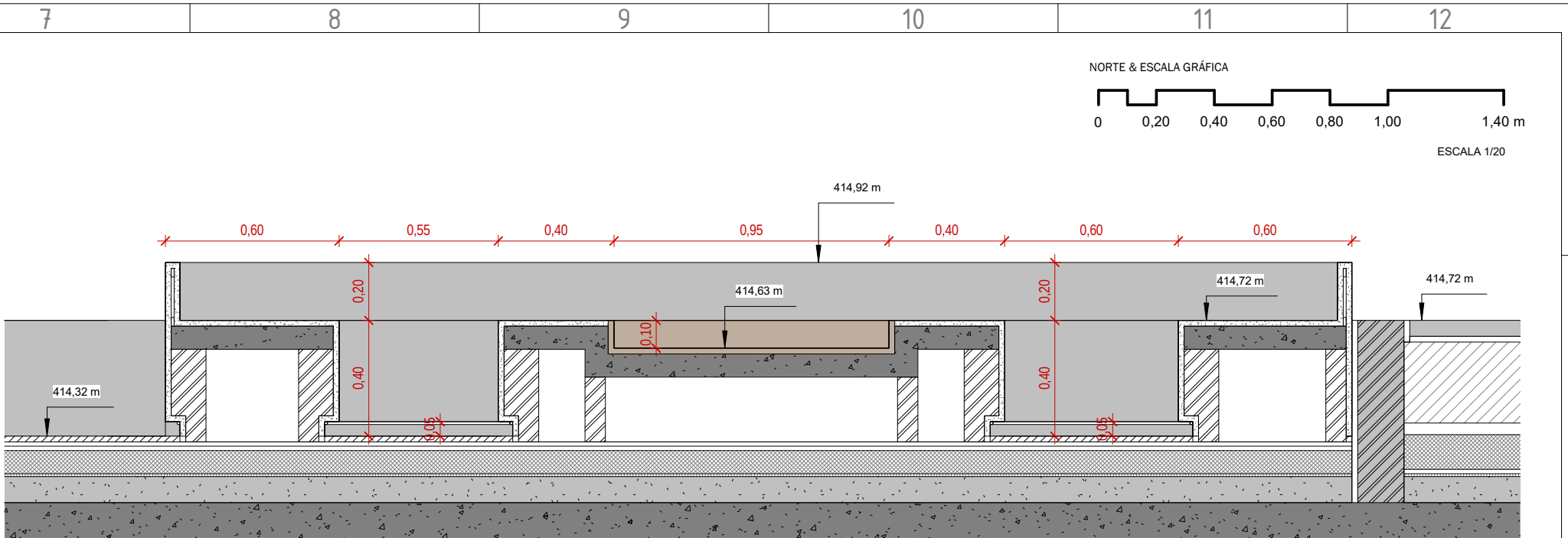
CORTE ESCALA: 1 : 20
