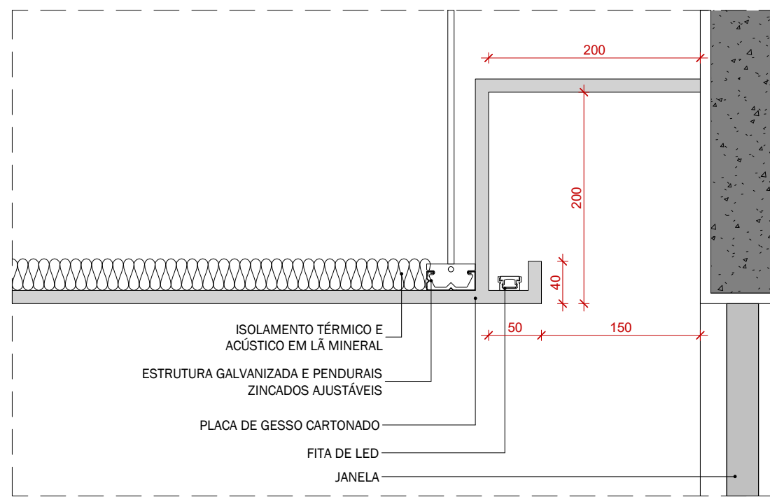
SNC 3 - SANCA DE LUZ - JANELA ESCALA: 1 : 5
