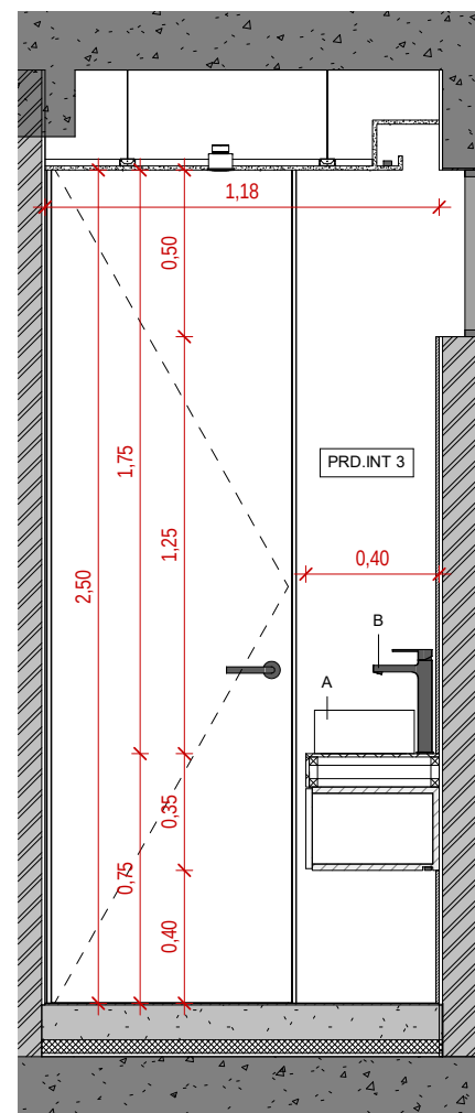
I.S. SOCIAL - CORTE AA ESCALA: 1 : 25
