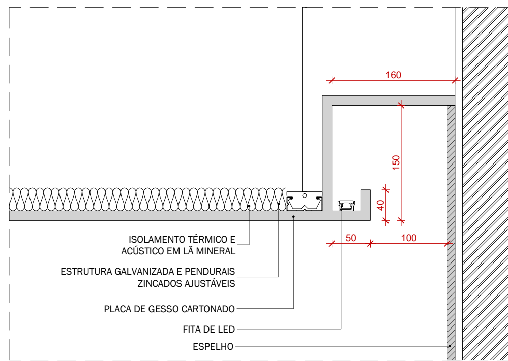
SNC 2 - SANCA DE LUZ - EСПEЛHO ESCALA: 1 : 5
