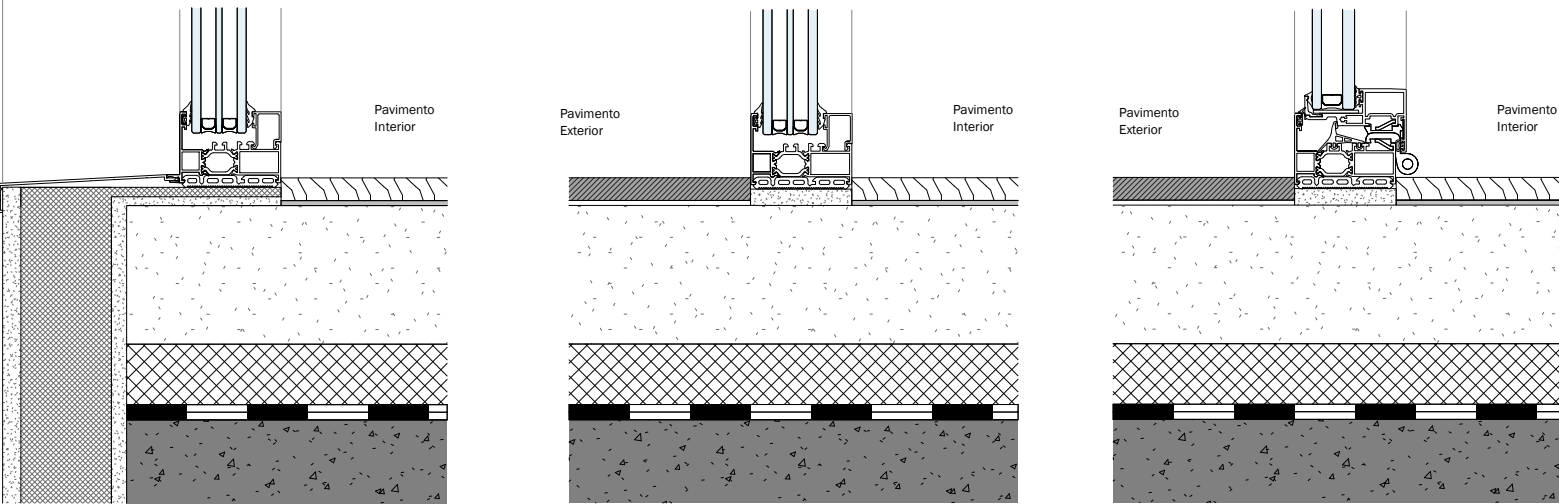
SOLEIRA 1 - LT OCULTO FIXO, COM KE 80
