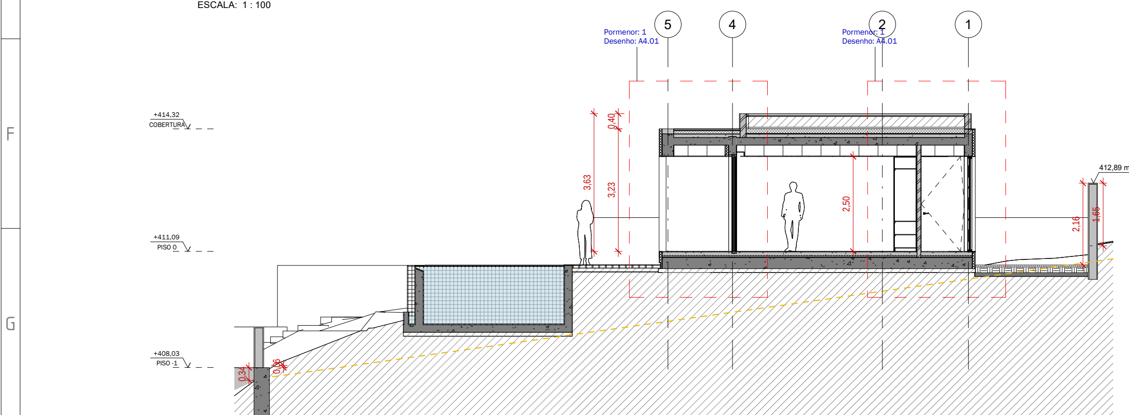
CORTE CC ESCALA: 1 : 100
