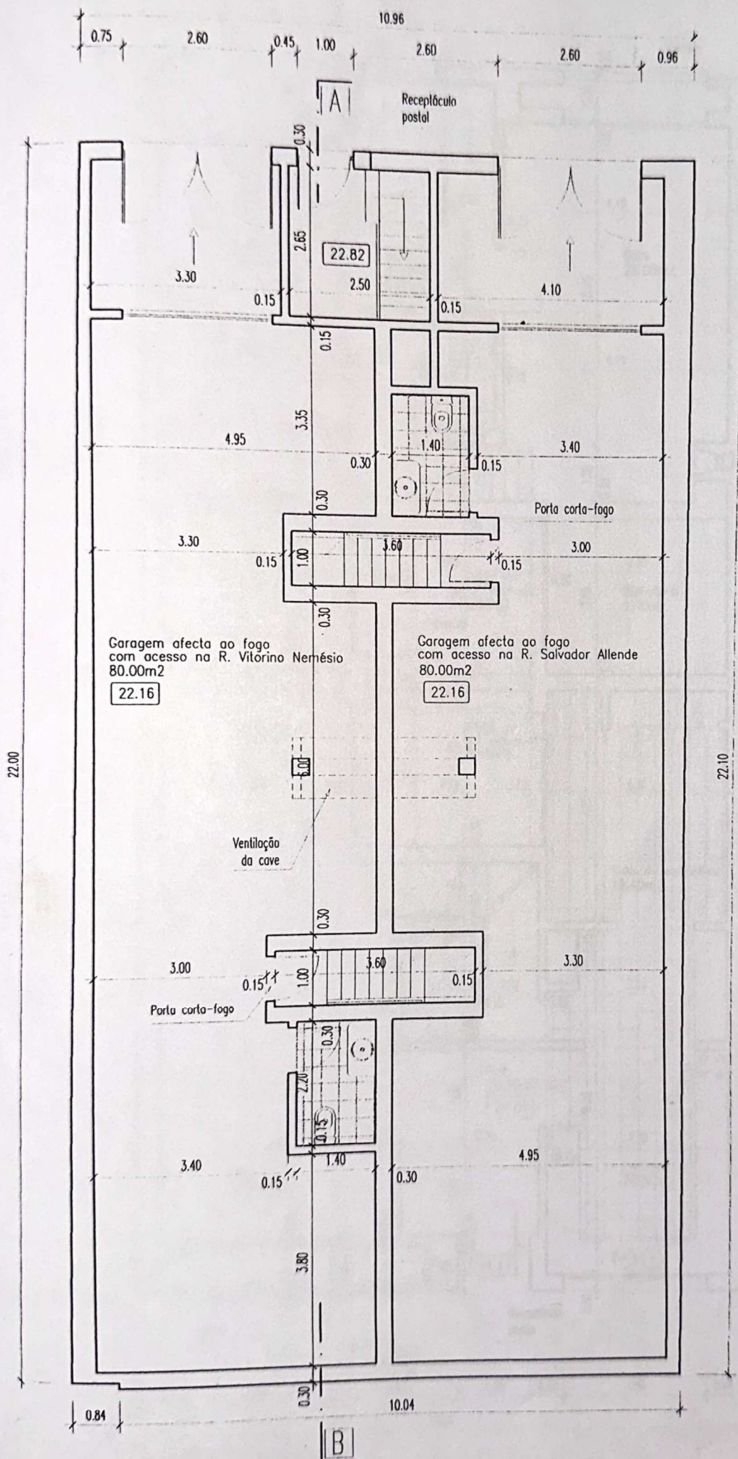
PLANTA - PISO -1
