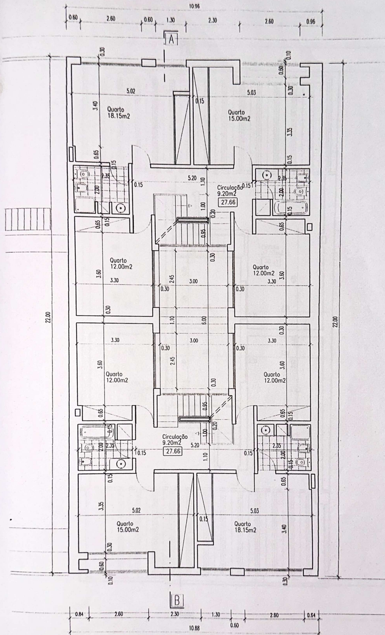
PLANTA - PISO 1
