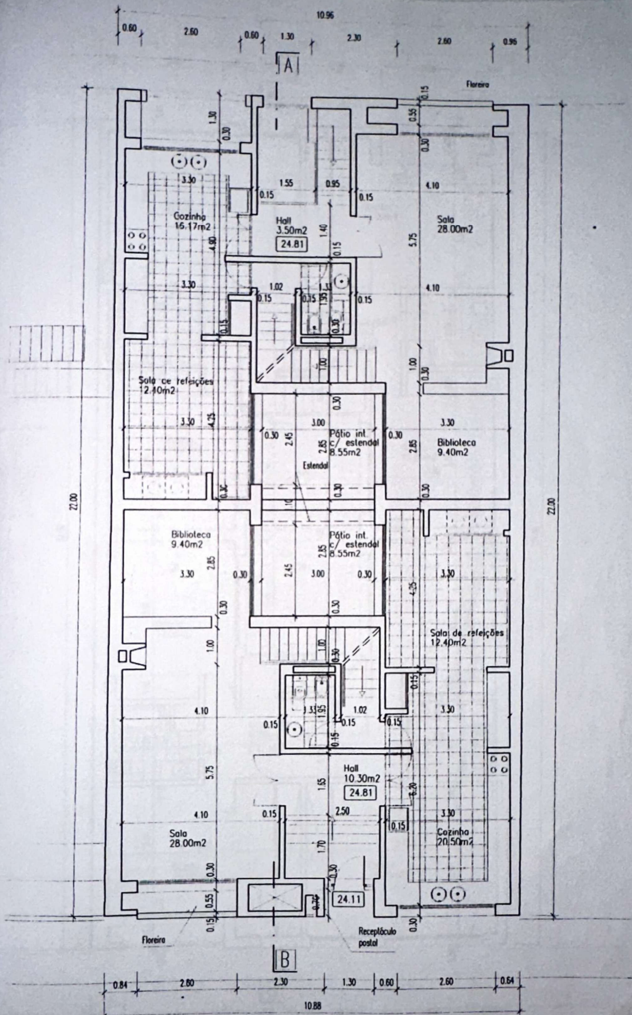
PLANTA - PISO 0
