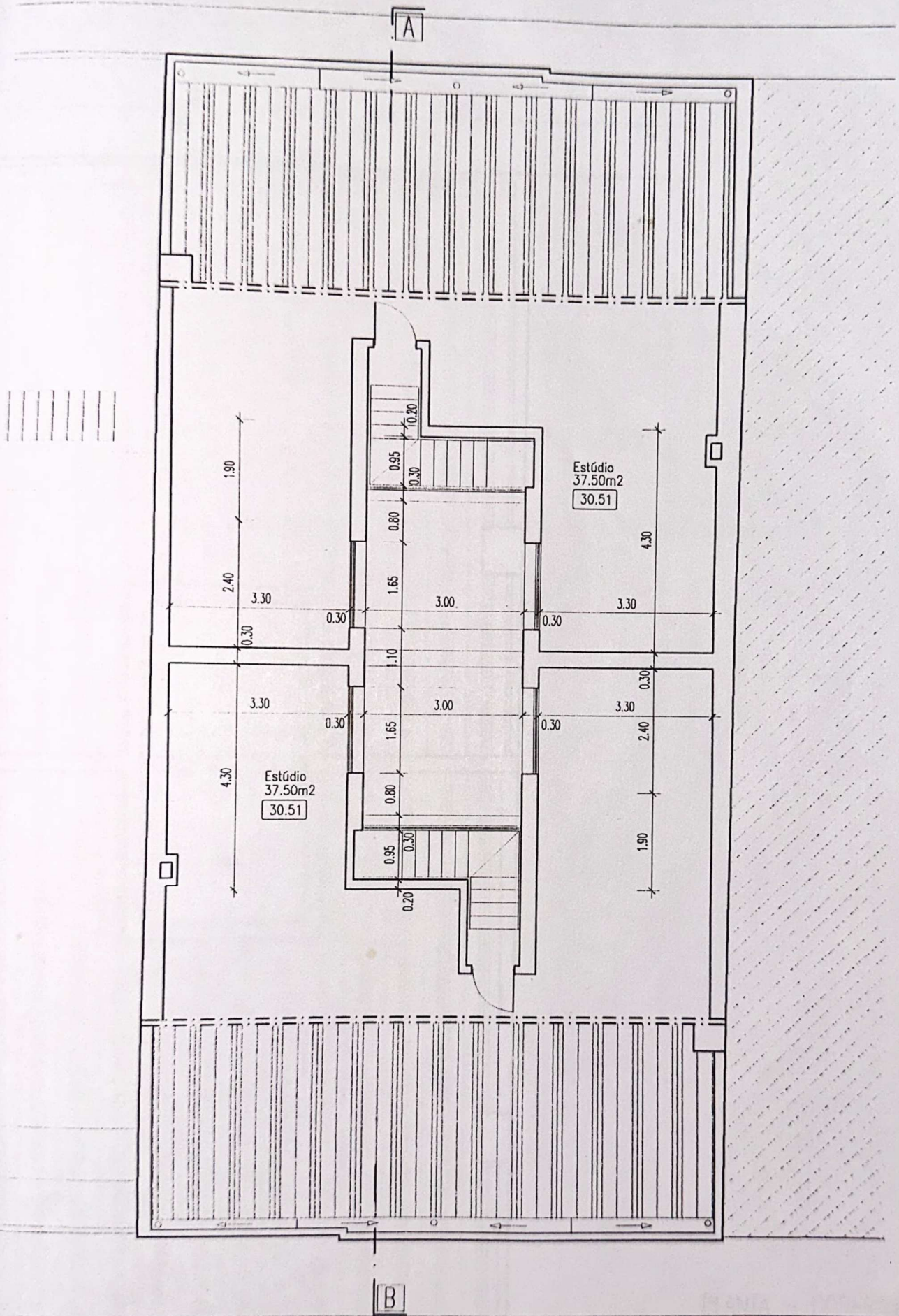
PLANTA - SOTÃO
