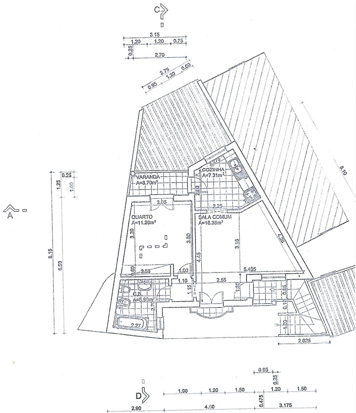
PLANTA DO 1º ANDAR (TELA FINAL)
