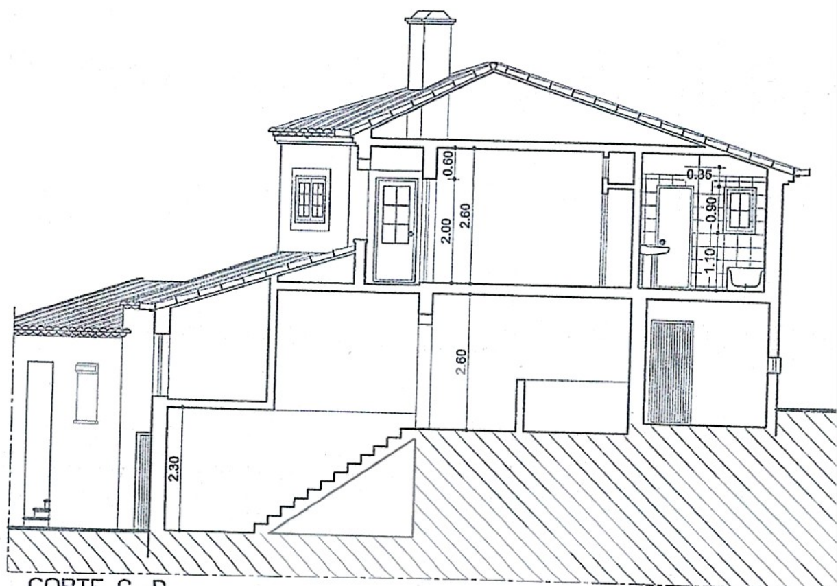
CORTE C-D
