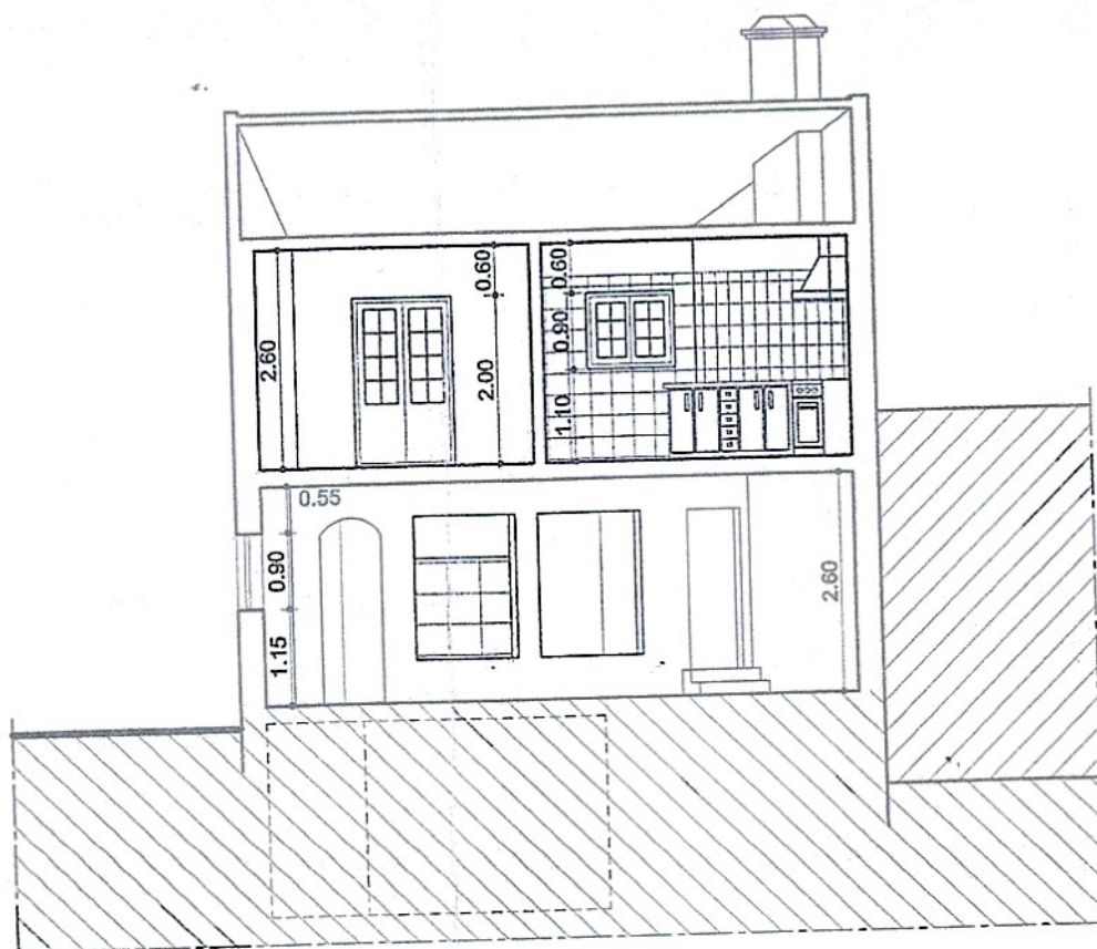
CORTE A - B
