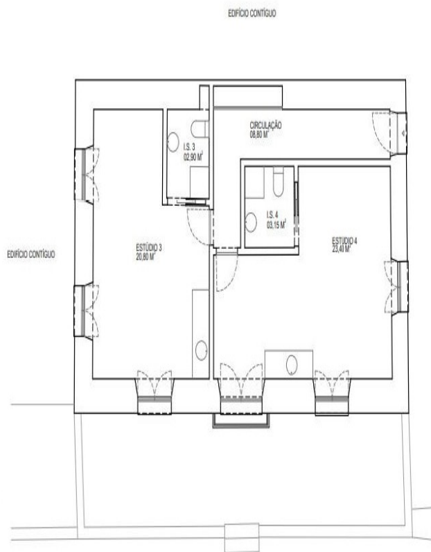
PLANTA DO PISO A COTA 21,47
