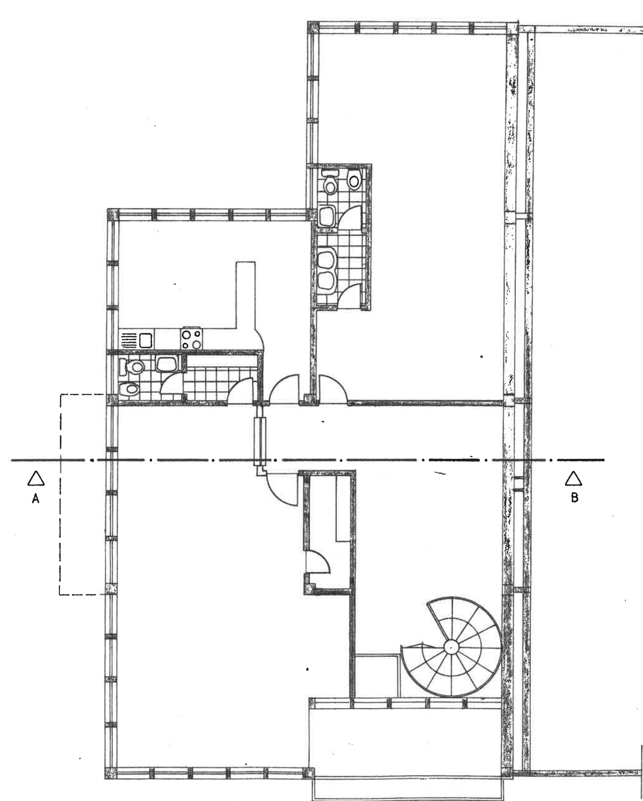
PLANTA DO ANDAR
