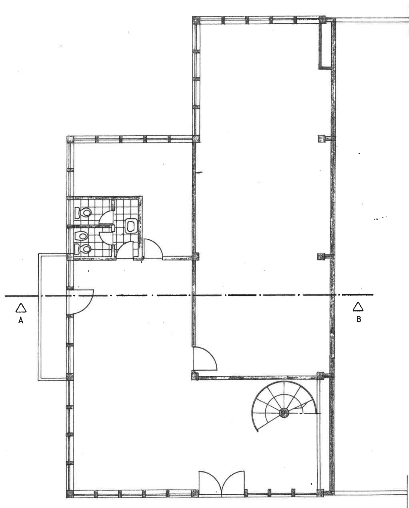
PLANTA DO RÉS-DO-CHÃO
