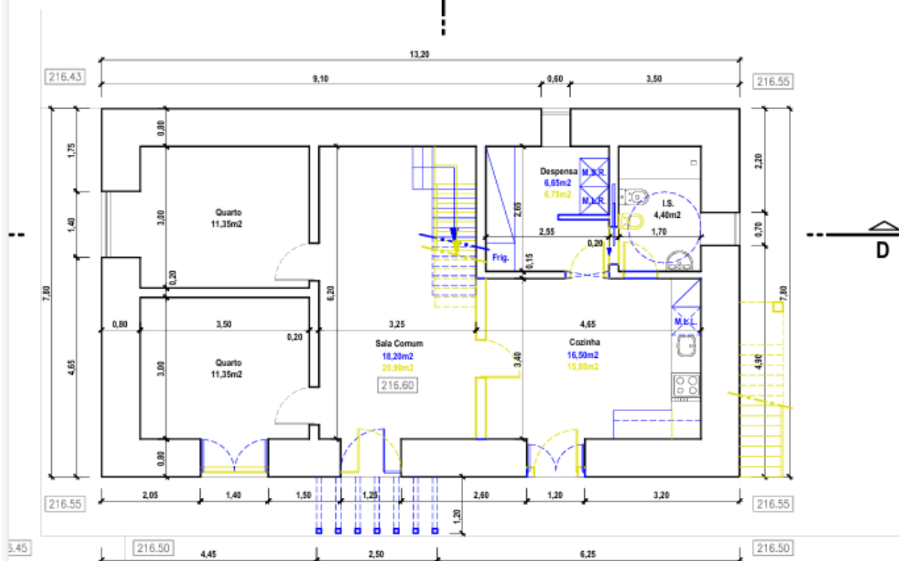
Planta do Piso - 102.95m 2
