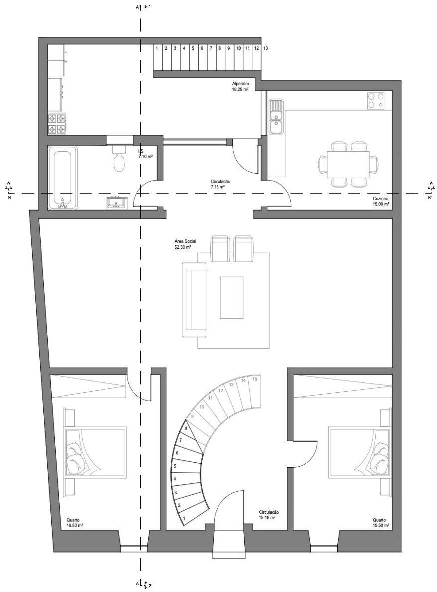
Planta - Piso 0
