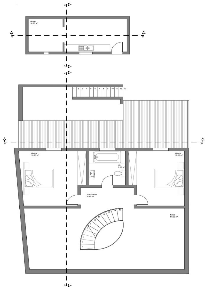
Planta - Piso 1
