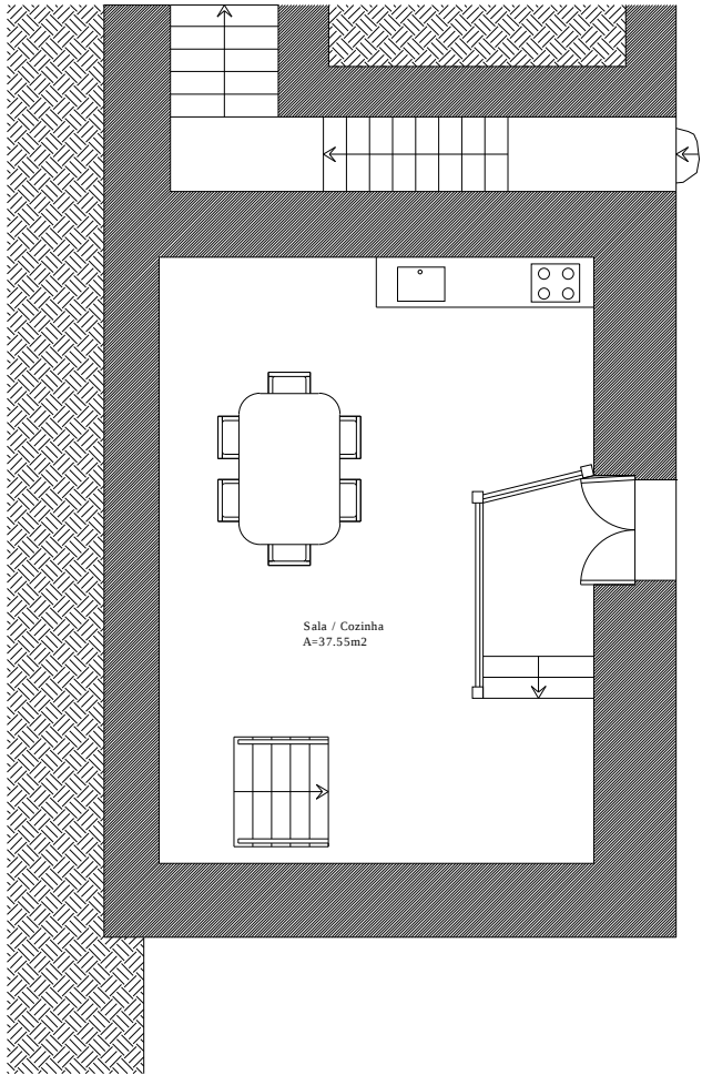
Planta do R/Chão Área de Construção - 60.00 m2
