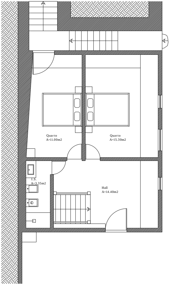
Planta do Piso 1 Área de Construção - 60.00 m2
