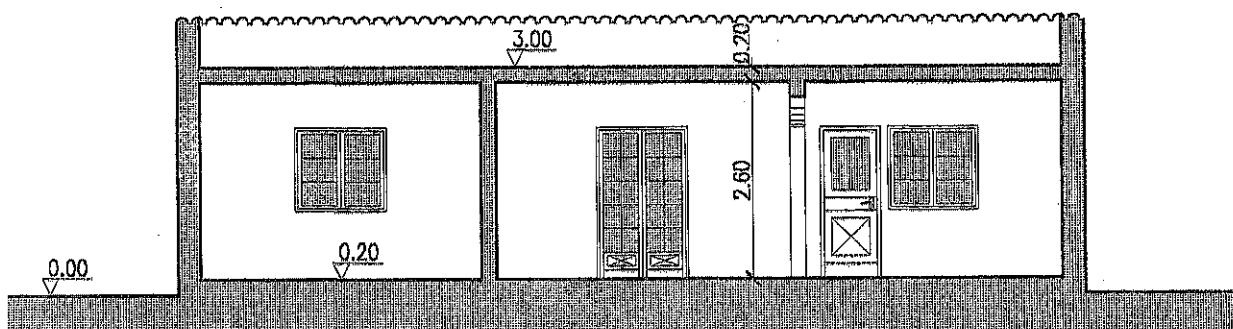
CORTE B-B
