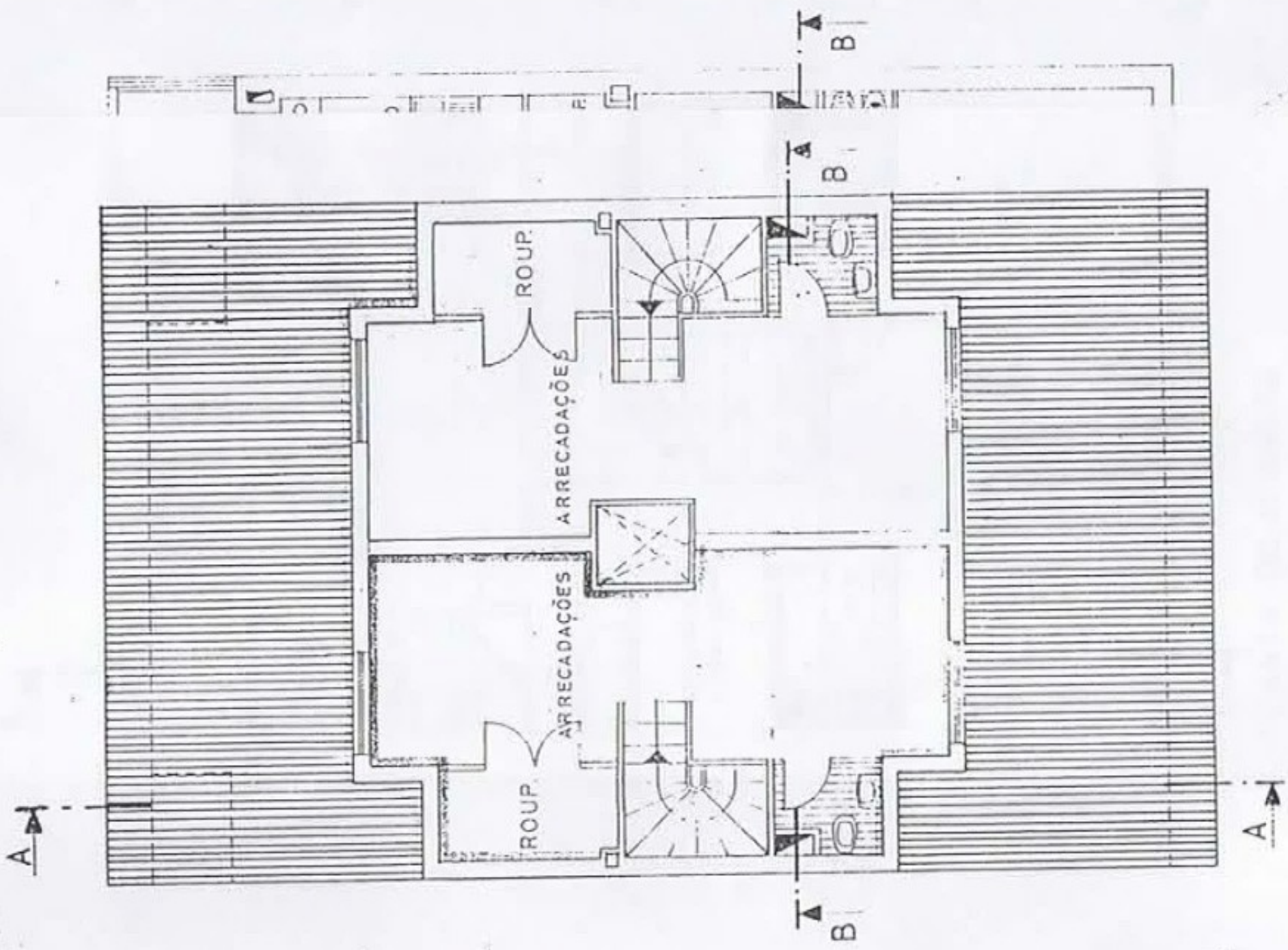
PLANTA DO SOTÃO
