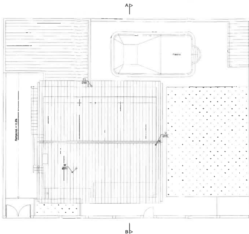
PLANTA DA COBERTURA
