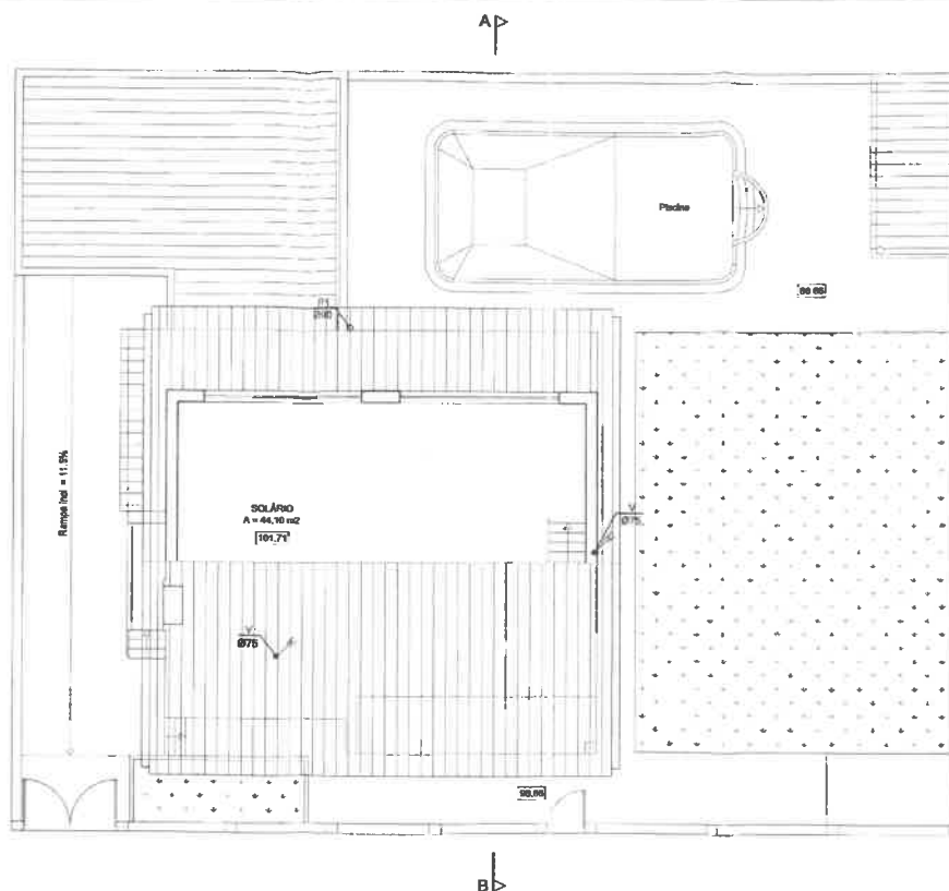
PLANTA DO SOLÁRIO
