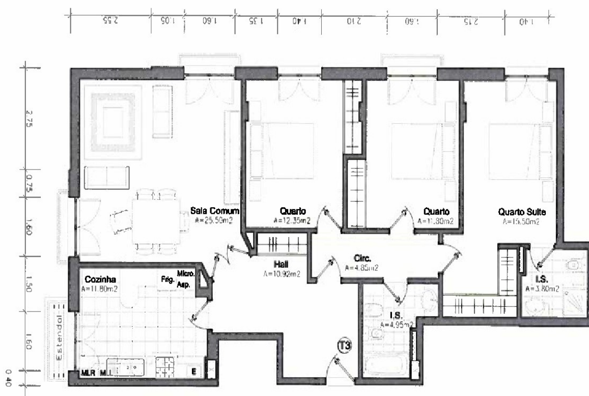
Planta simplificada da habitação Apartamento - Tipologia T3 - Dir.º (4 Assoalhadas)
