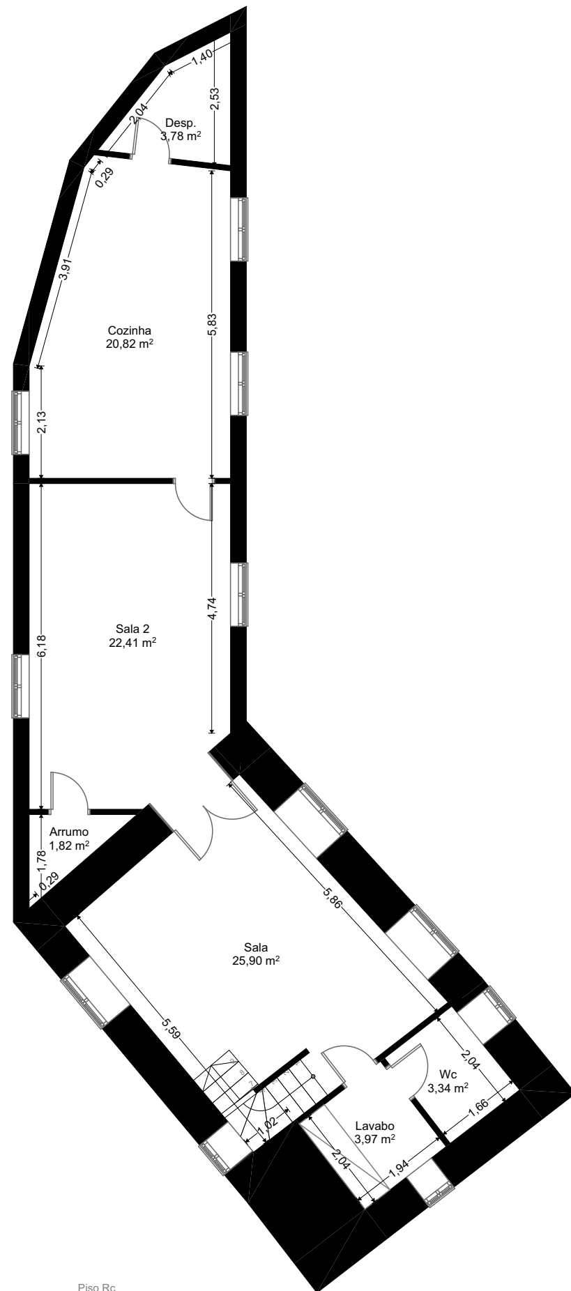
Piso Rc
