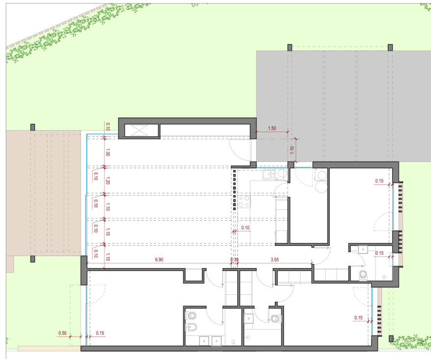
PLANTA DO TECTO
