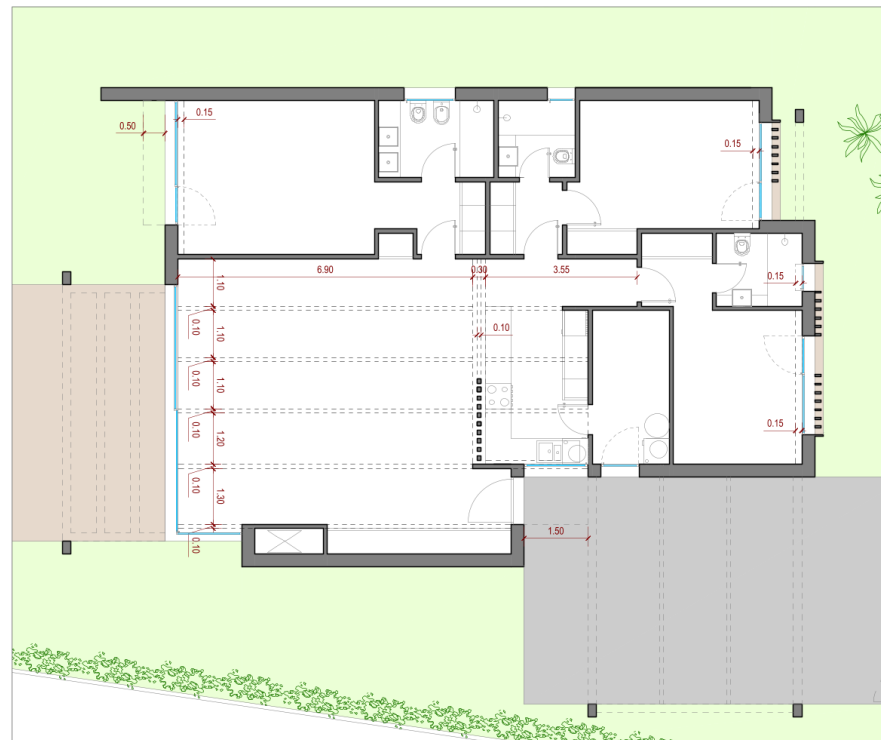
PLANTA DO TECTO
