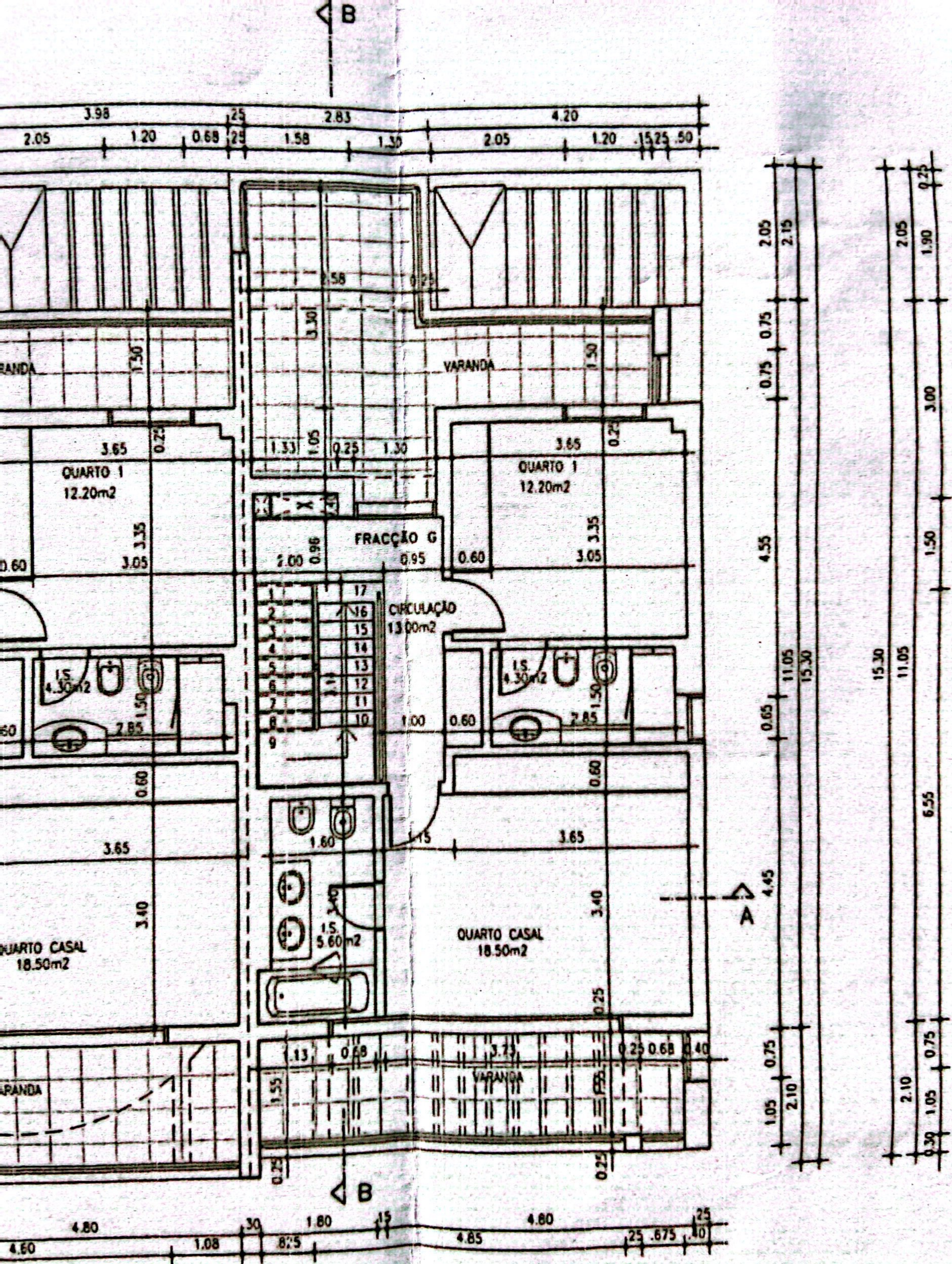
PLANTA DO 1º ANDAR
